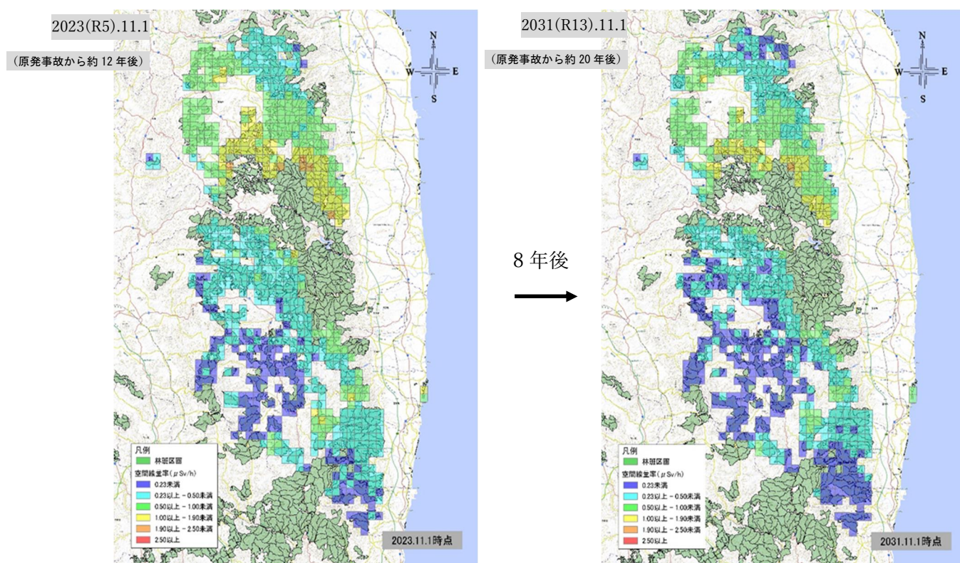
国有林内空間線量率の将来予測（2023年から2031年）
