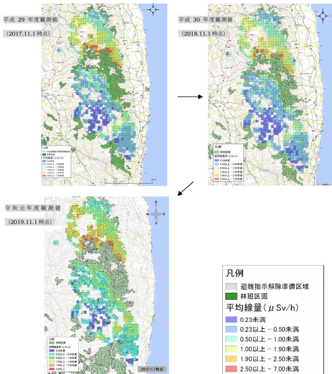
図 2.1 国有林内空間線量率の推移
