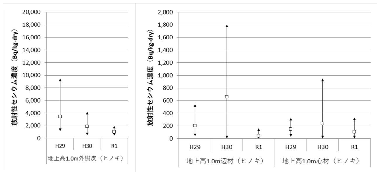
図 4.1 ヒノキにおける放射性セシウム濃度* 3
