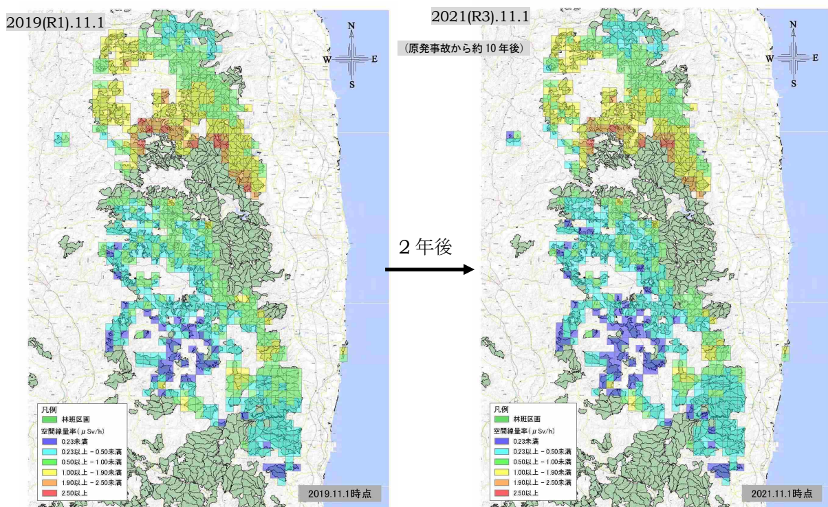
図 3.1 国有林内空間線量率の将来予測（2019 年～2021 年）
