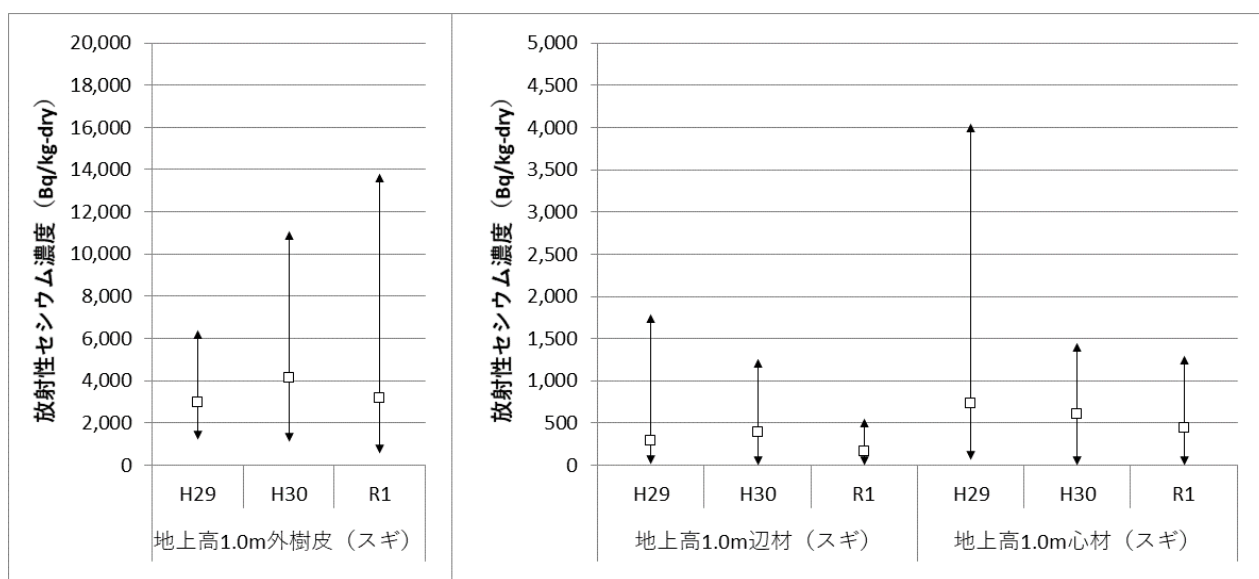
図 4.2 スギにおける放射性セシウム濃度* 3
