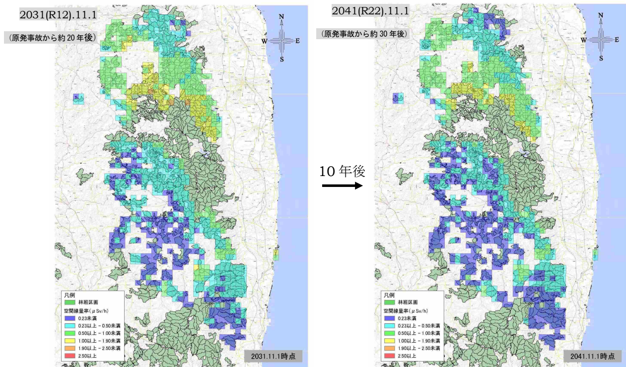
図 3.2 国有林内空間線量率の将来予測（2031 年～2041 年）
