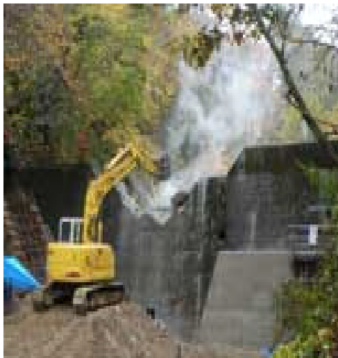
図4．防災と溪流環境復元のため、治山ダムの中央部撤去の様子（平成21年10月実施）
