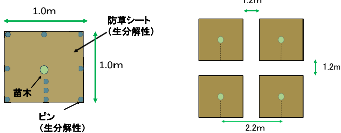
図1.防草シートの固定
