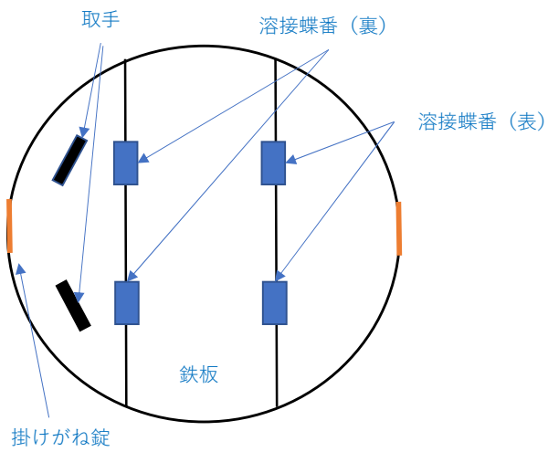
蓋横断面図
