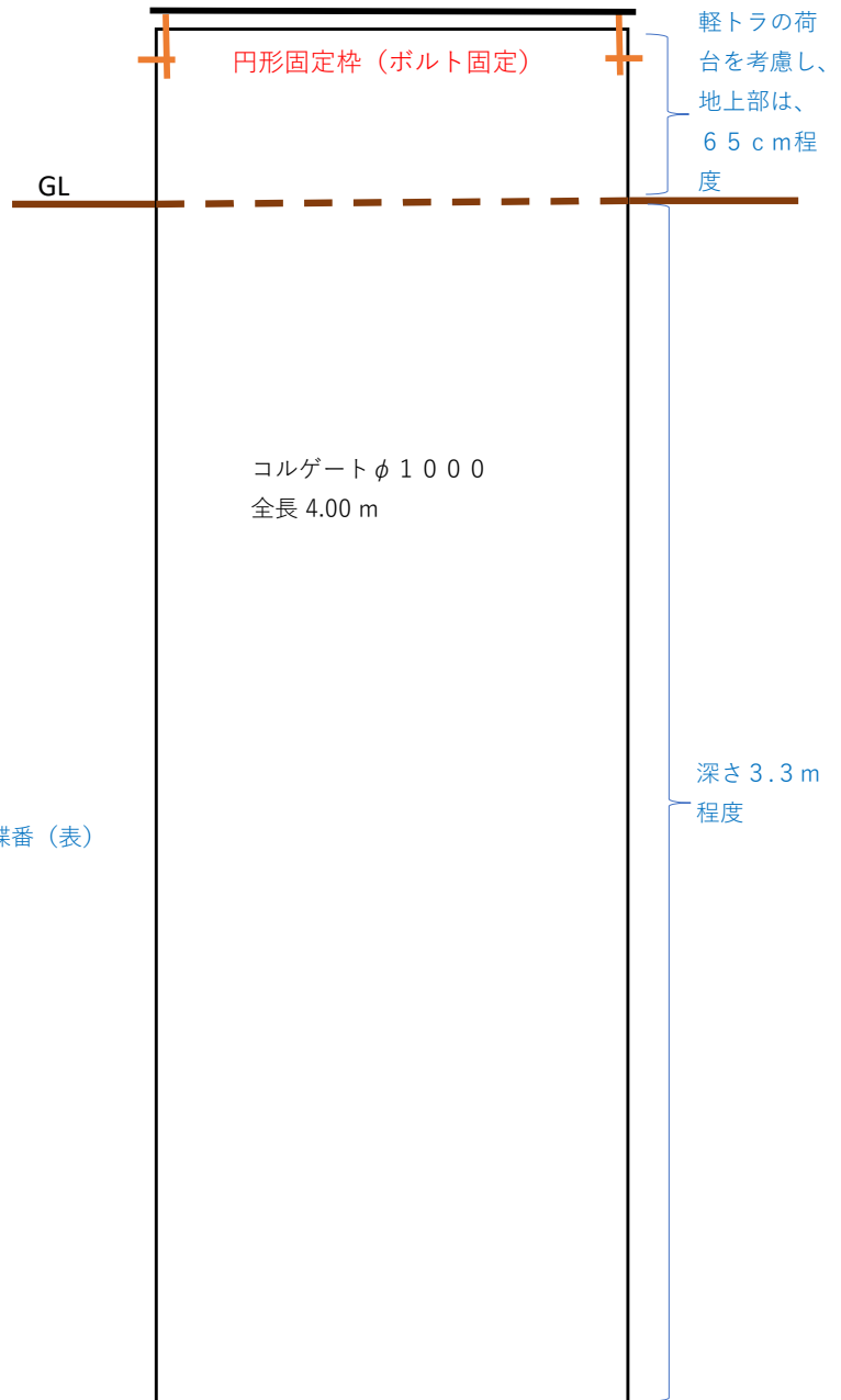
断面図
