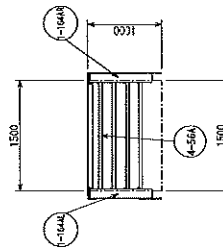
断面図 (C-C矢視) (単位: mm)
