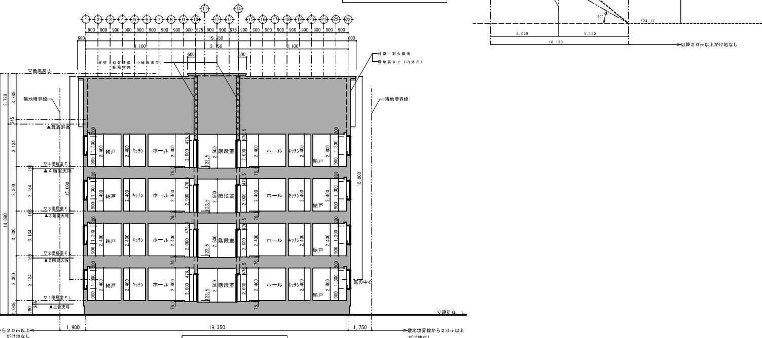
南北 断面図 S=1/100
