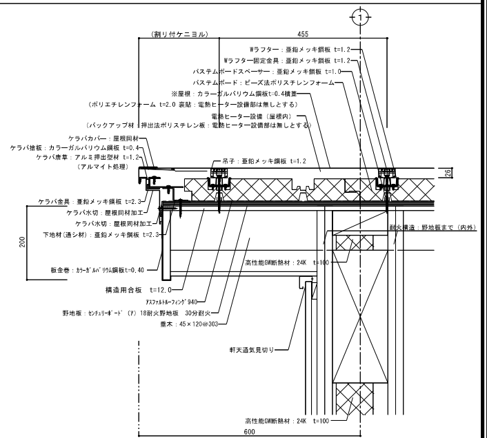
ケラバ（電熱ヒーター設備部）
