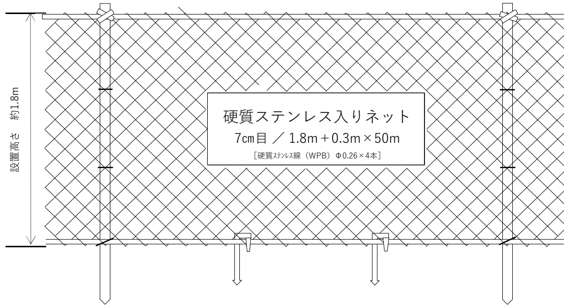
正面図
