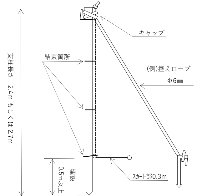
補強部 (例)
