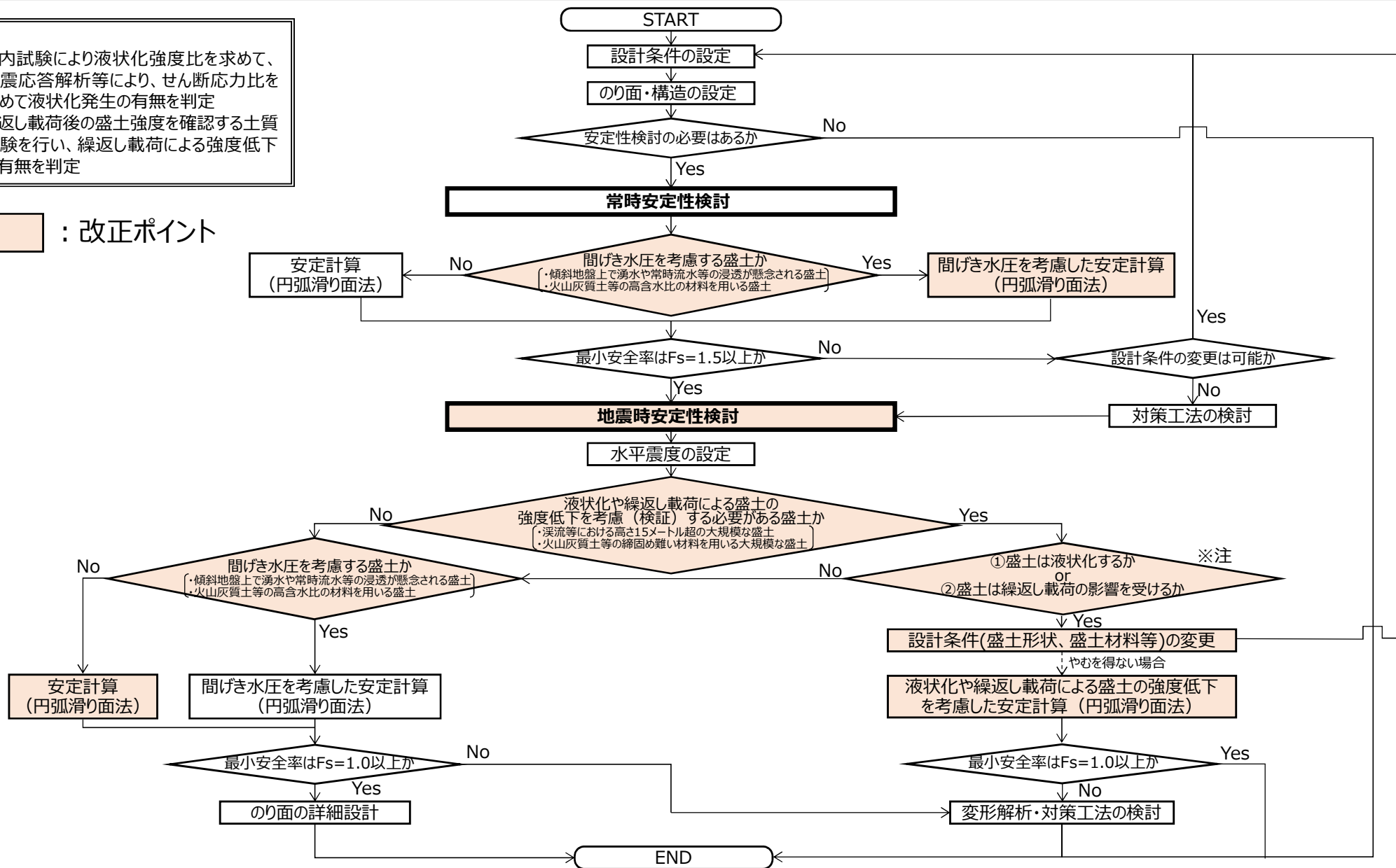
図 盛土のり面の一般的な安定検討フロー
