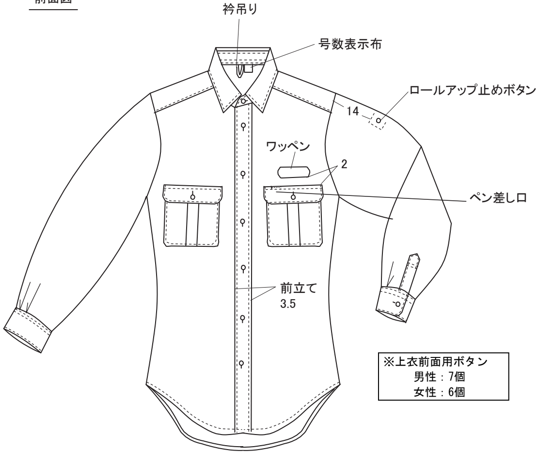
前面図
