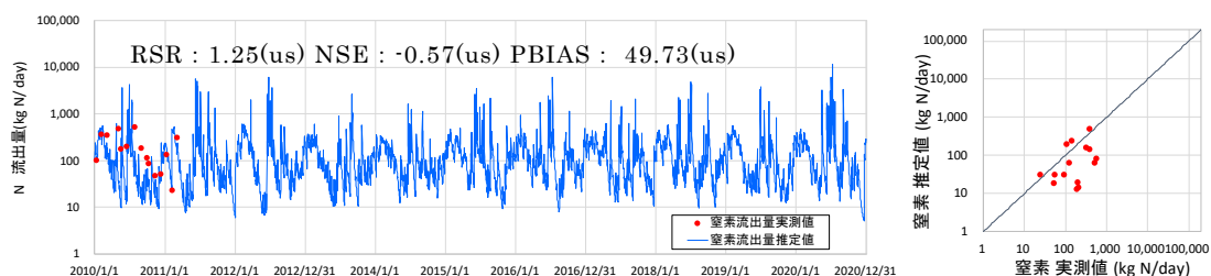
図 V-24 五木宮園におけるハイドログラフ (窒素)
