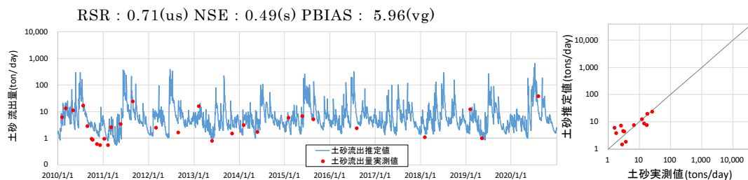
図 V-25 柳瀬におけるハイドログラフ (SS)
