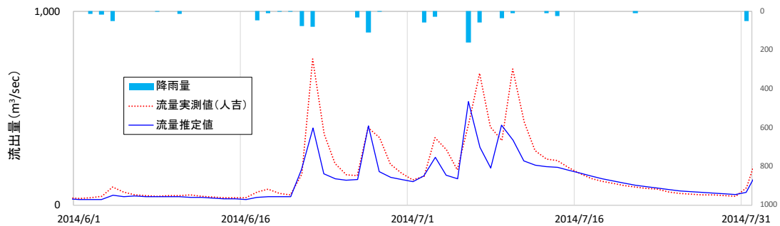
図 V-18 人吉における出水時のハイドログラフ
