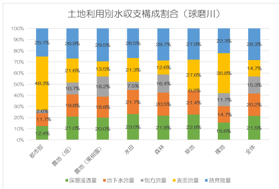
図 V-9 土地利用区分別の水収支における構成割合
