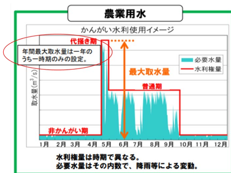
図 V-6 農業用取水量設定のイメージ
