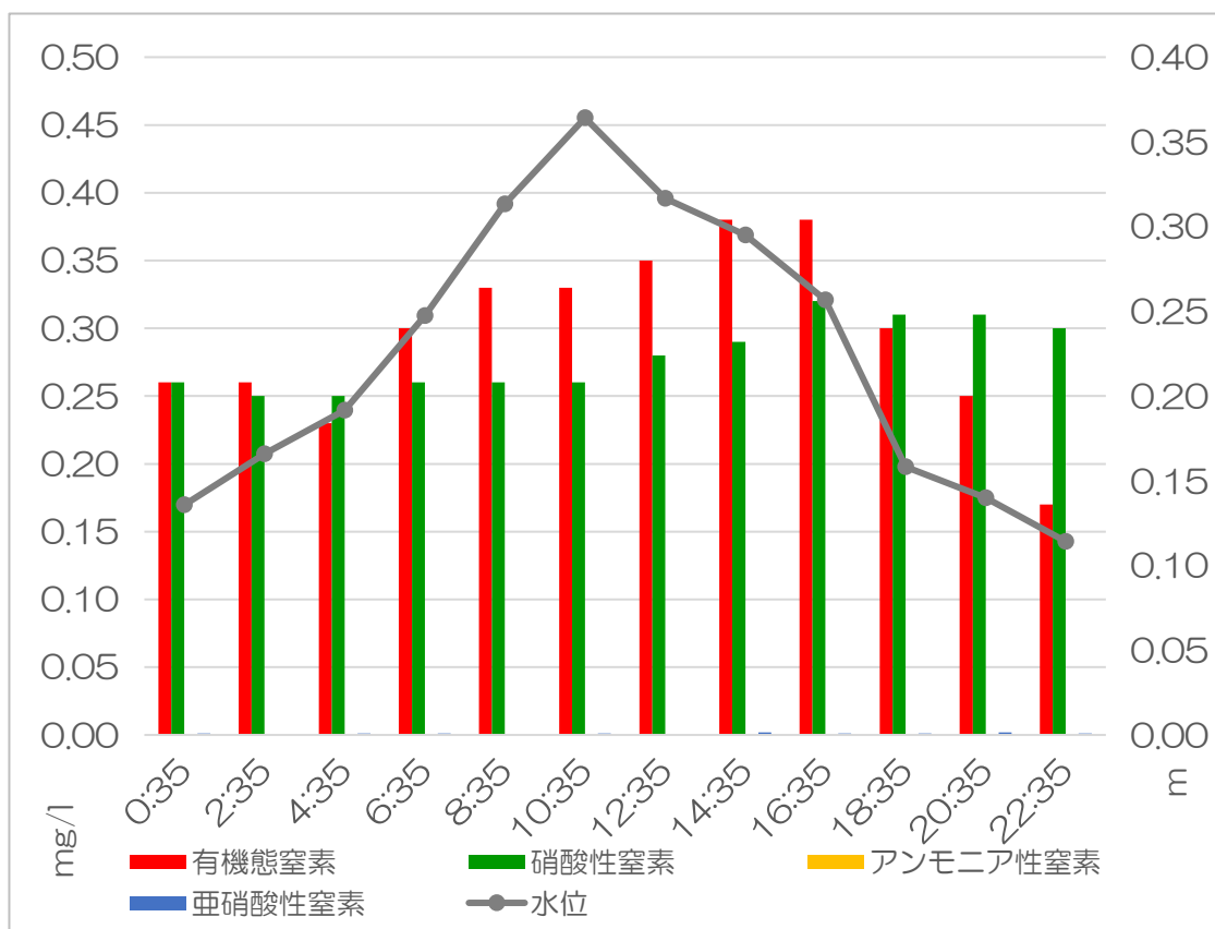
図 IV-9 推定される水位と窒素化合物の関係
