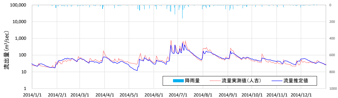
図 V-17 人吉における一年分のハイドログラフ（2014 年）
