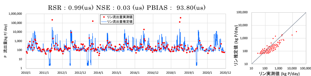
図 V-32 横石におけるハイドログラフ (リン)
