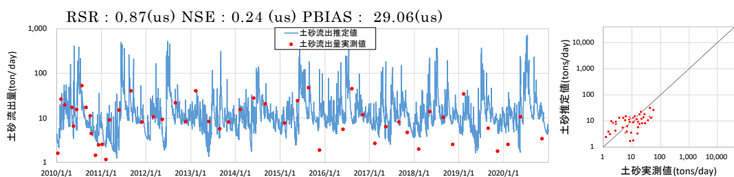
図 V-28 人吉におけるハイドログラフ（SS）
