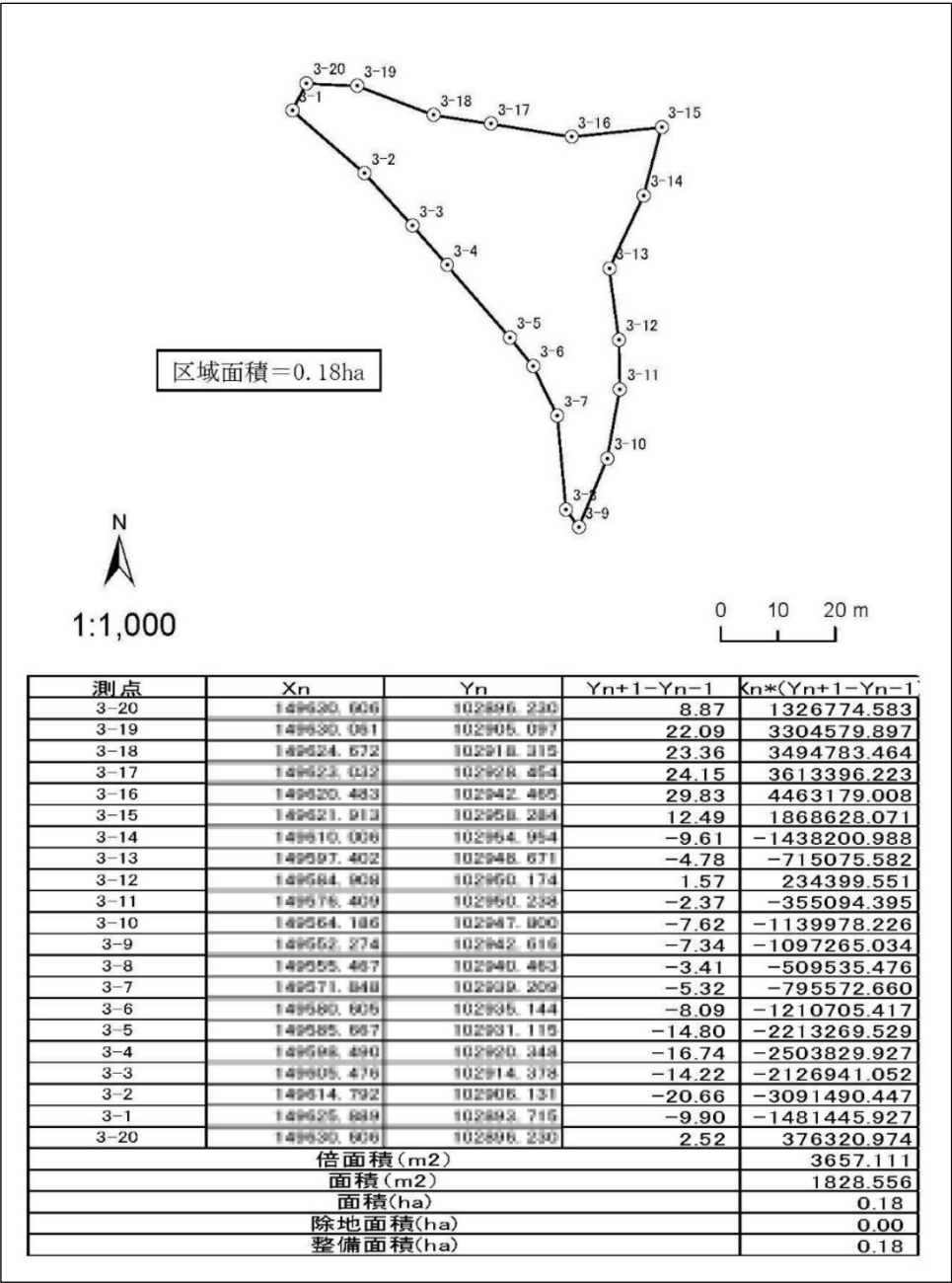
図 5-4 周囲測量成果の例
