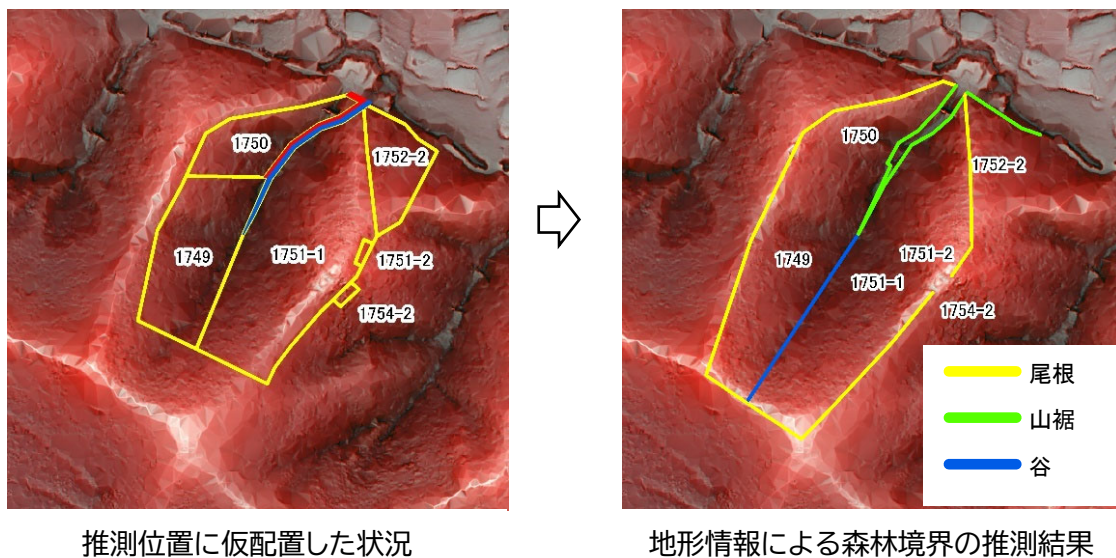
図 5-7 地形情報による森林境界の推測例
