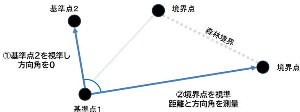
図 8-1 現地での座標取得
