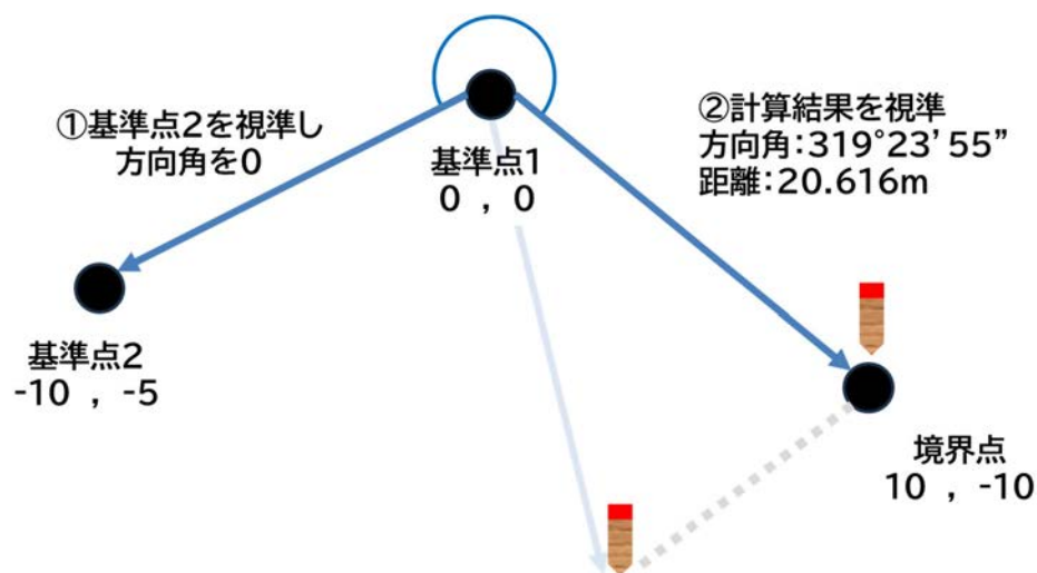
図 8-2 復元測量の計算方法
