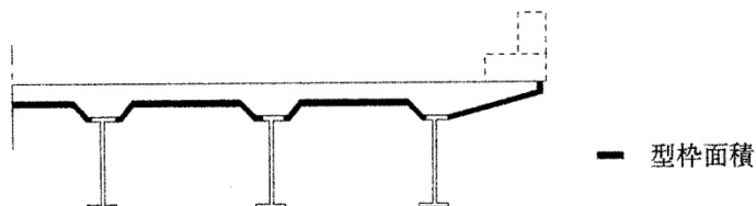
図2-2 標準床版断面
