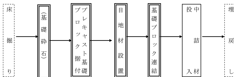
図2-2 施工フロー
