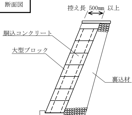
断面図
