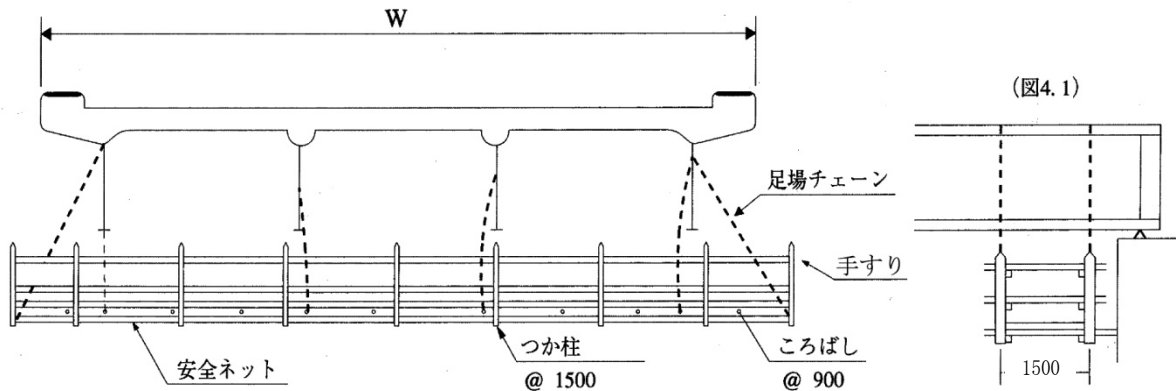
図3.3 橋脚回り吊足場
