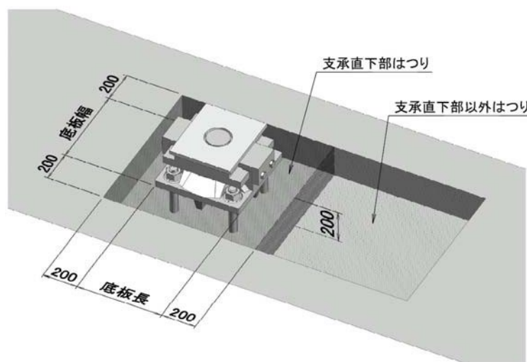
図3. 2 参考図 (沓座コンクリートはつり)
