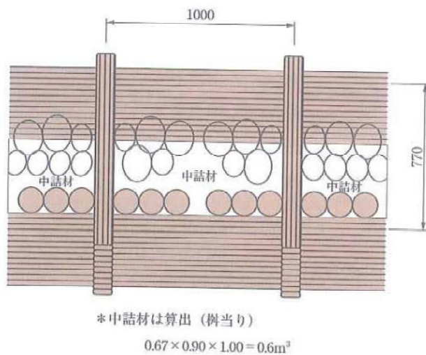
3分法型平面図
