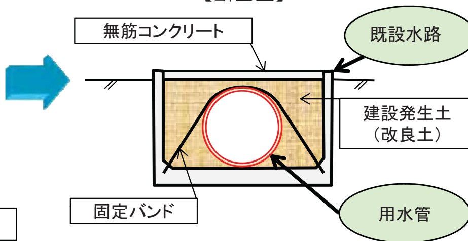
水路内敷設状況
