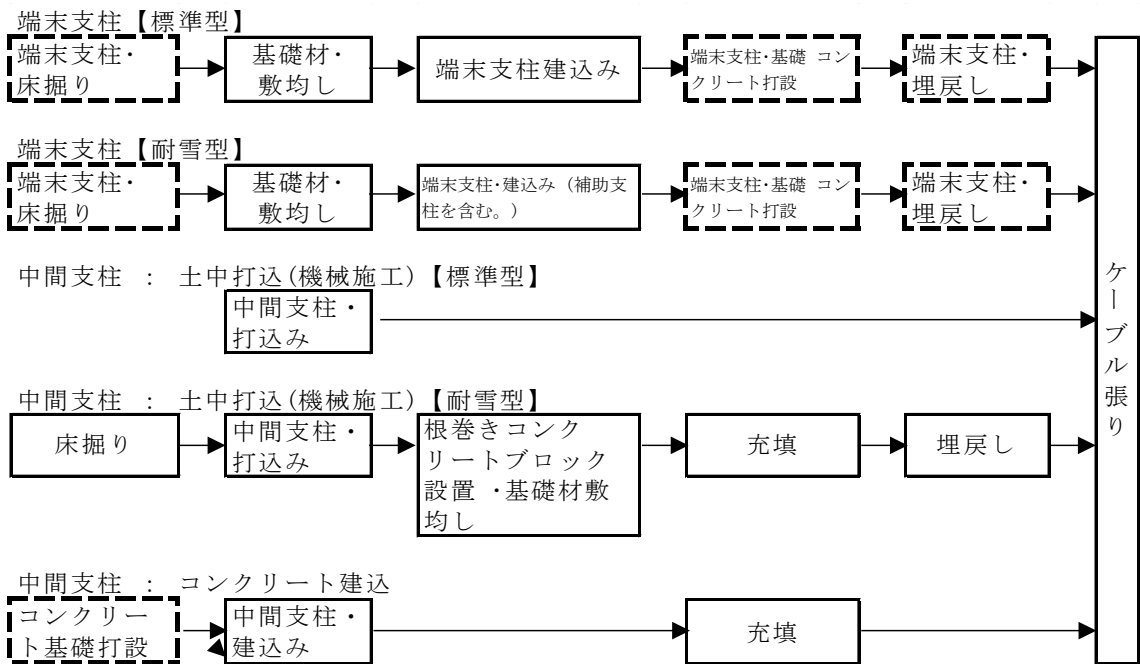
図 2-1 施工フロー
