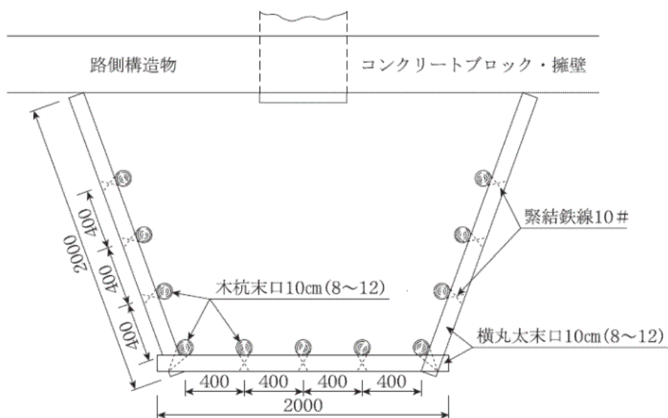
〔平面図〕
