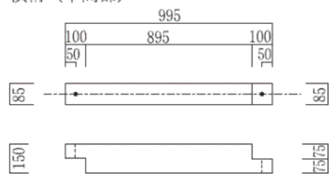
横桁（中間部）
