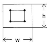
(4本配筋の例)
