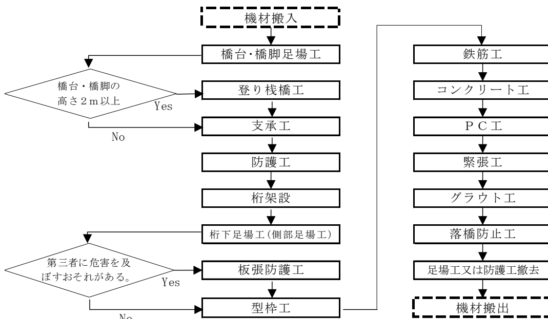
図 2-1 施工フロー
