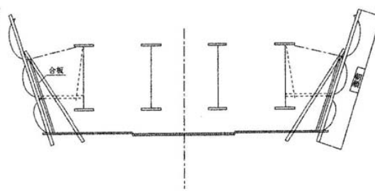
シート防護 (含朝顔)
