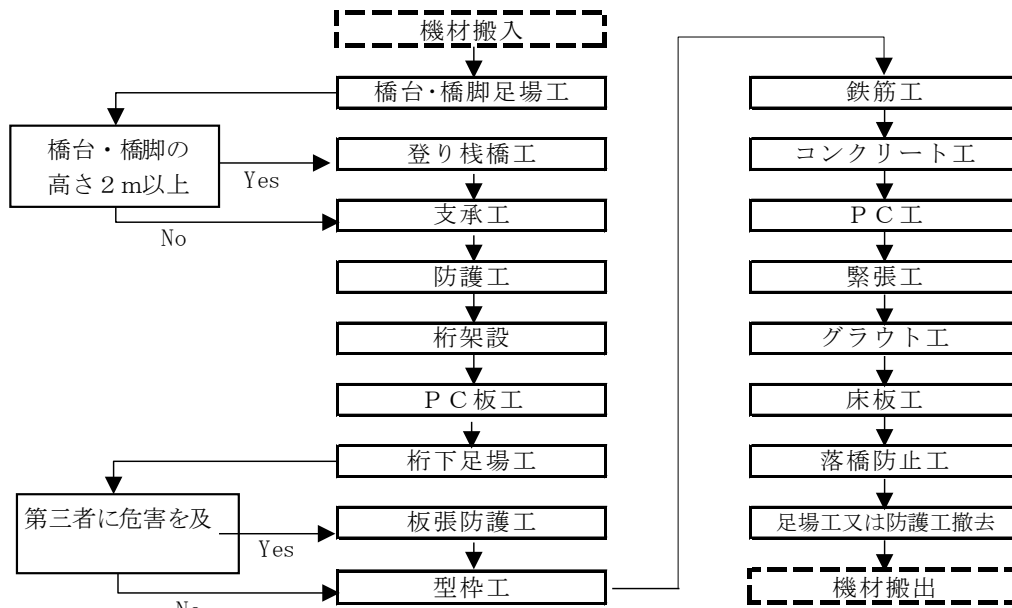
図 2-2 施工フロー(PCコンポ桁)
