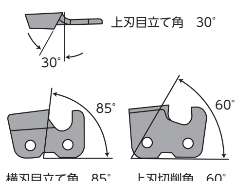
図6-16 マイクロチゼル型
