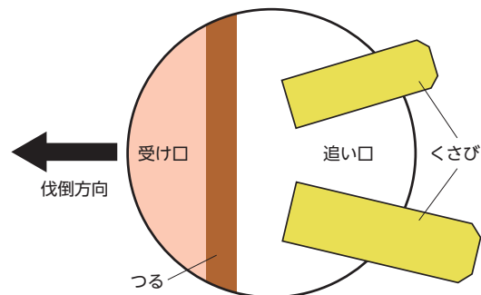
図 17-14 くさびを正しく使い、確実な伐倒を行う
