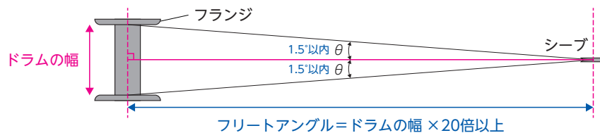
図7-6 ドラム幅の20倍以上の距離にシーブ(滑車)を設置する —フリートアングル
