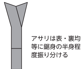
図5-13 アサリは刃先を少し曲げる程度
