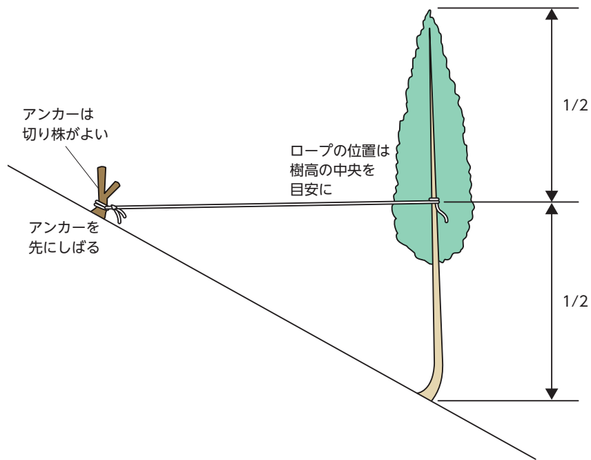
ず ゆきお ほうほう 図10-17 雪起こしの方法
