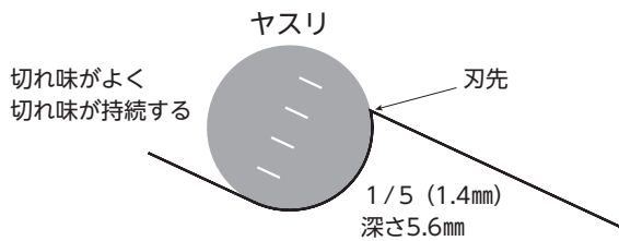
図5-11 刈刃と丸ヤスリの関係 丸ヤスリで、径の1/5が刃の外側に出る程度で目立てするのがベスト。
