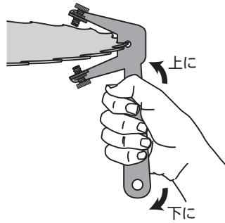
図5-12 この原理で歯先を曲げる「アサリ割り器」の例
