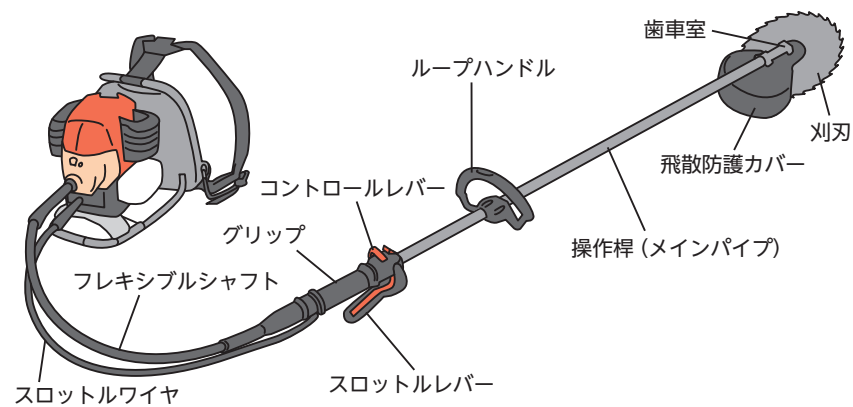
ず せおいしきかりはらいき 図5-2 背負式刈払機
