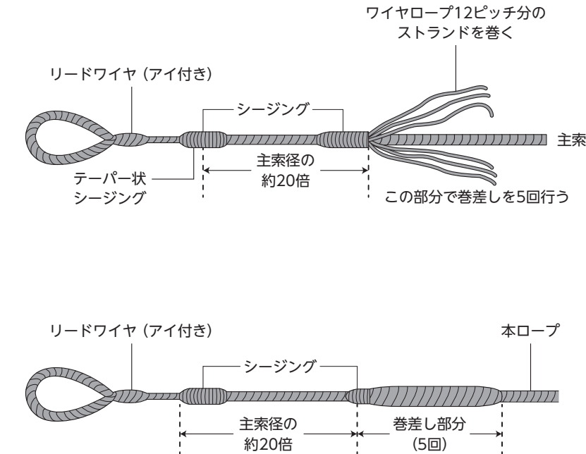
図7-14 ベケット加工方法
