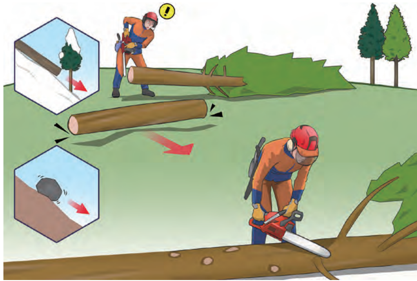
図15-3 上下作業の禁止
