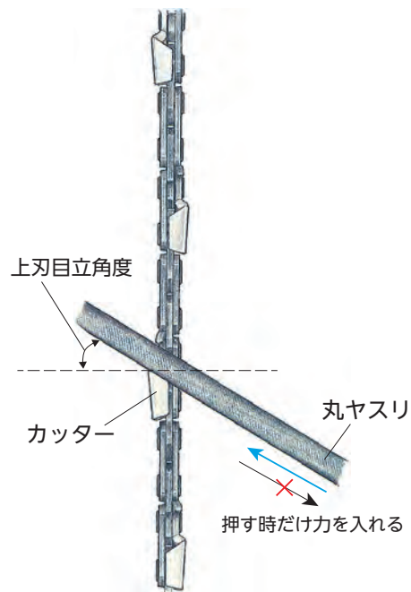
図6-19 丸ヤスリの当て方
