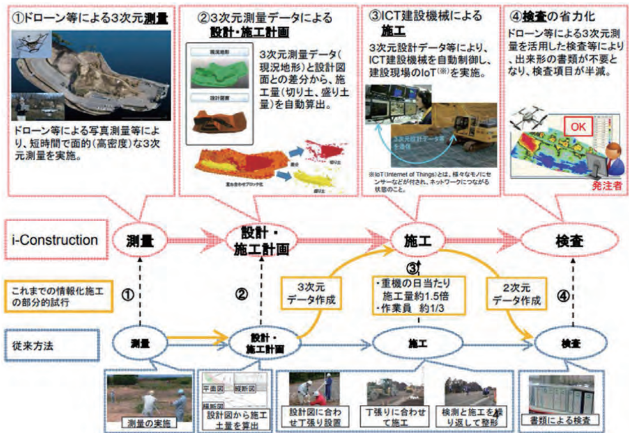
図2-1 i-ConstructionにおけるICT土工の例
