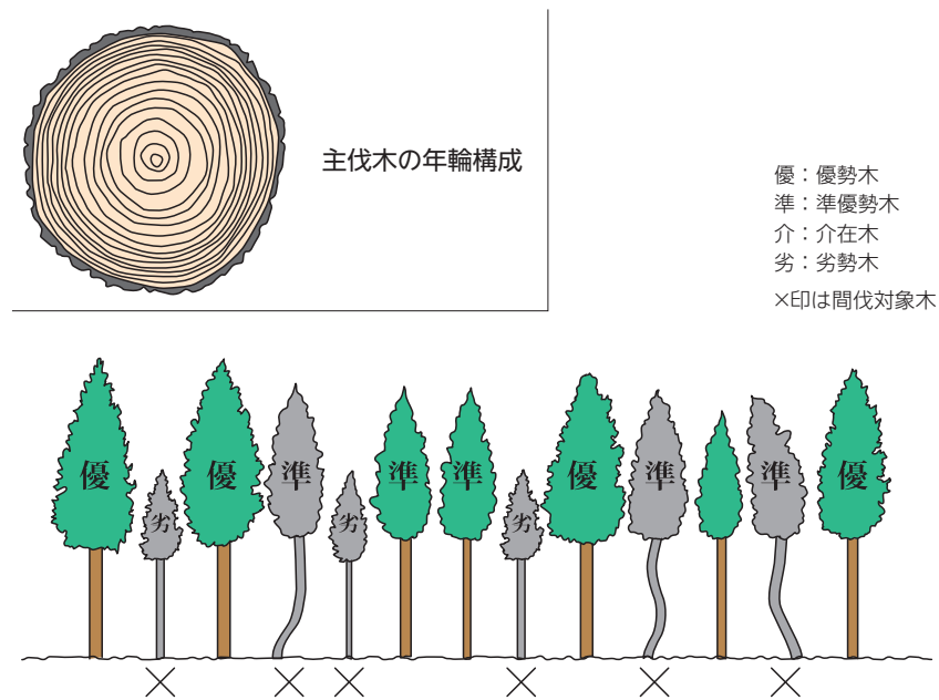
ず 図14-11 下層間伐
