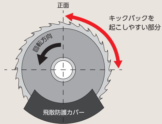
キックバックを起こしやすい部分
