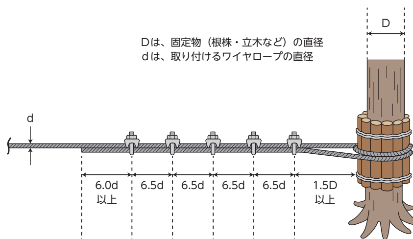
ず ど ほうほう ねかぶ と つ 図7-9 クリップ止めの方法(根株などへの取り付け)
