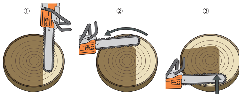
図13-11 材がガイドバーの長さよりも大きい場合(両持ちの材)
