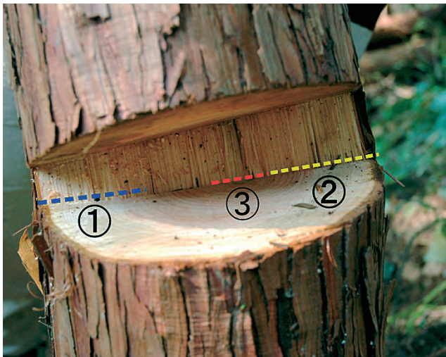
図19-13 つるの処理の例—かかり木を回転させる場合
