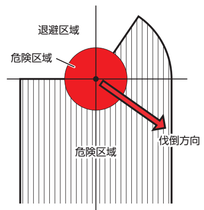
図 15-14 退避場所を決定する
