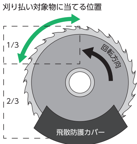
図10-12 草類の刈り払い位置
