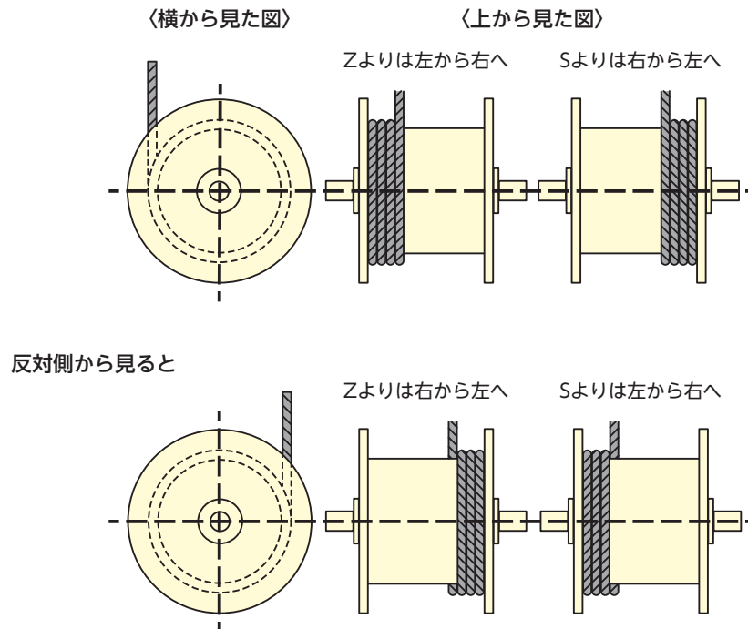
図7-5 集材機などのウインチドラムへの巻き方
