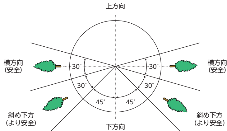
図17-3 安全な伐倒方向
