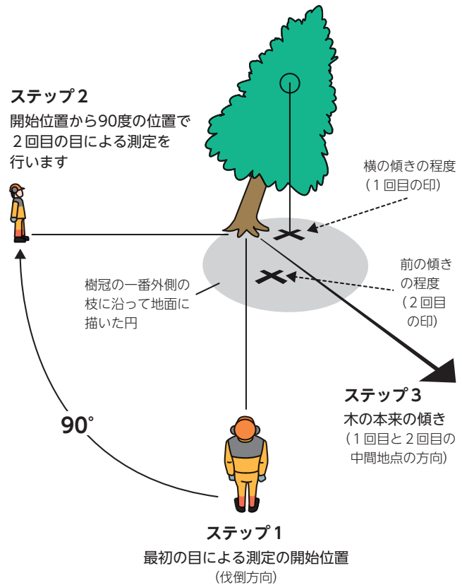
図 17-2 木の傾きを測定する
