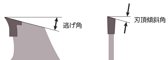
図5-15 チップソーの目立て角度の例 逃げ角は10~15度。メーカーの取扱説明書を参考にします。
