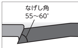
写真5-2 なげし角
