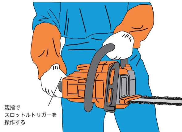
図 15-8 水平切りの時の持ち方
