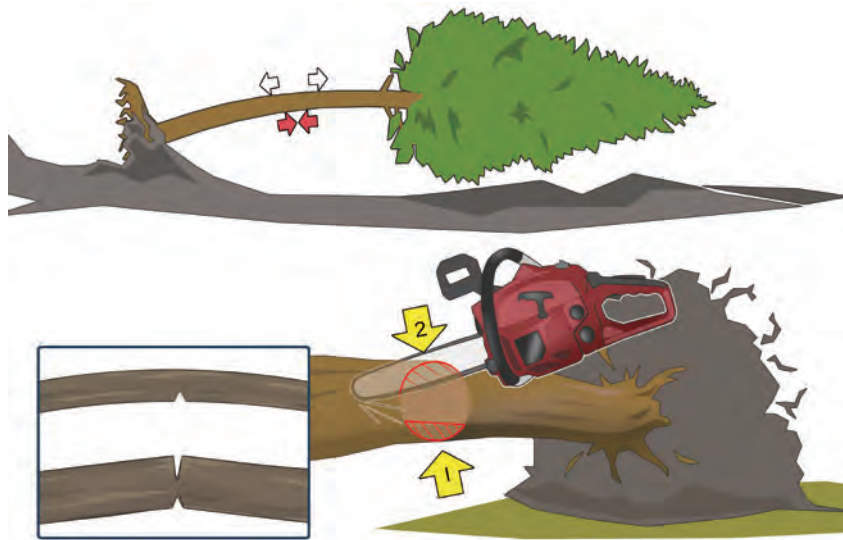
図19-21 極度に曲がっている木の切り離し方法 極度に曲がっている時は、曲がりの内側に切り欠きをします。
