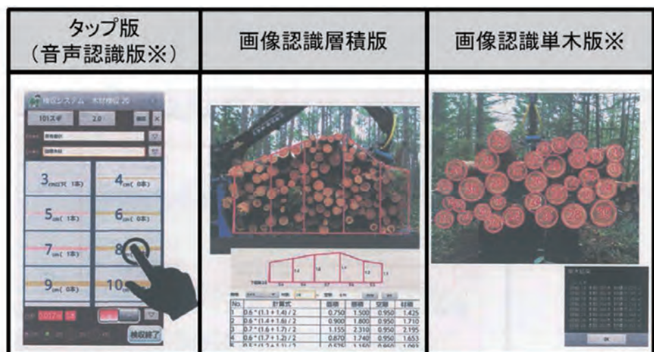
図2-11 スマホアプリを使った木材検収システム
