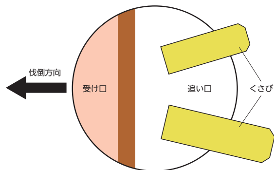
図15-18 くさびの打ち込み位置の例
