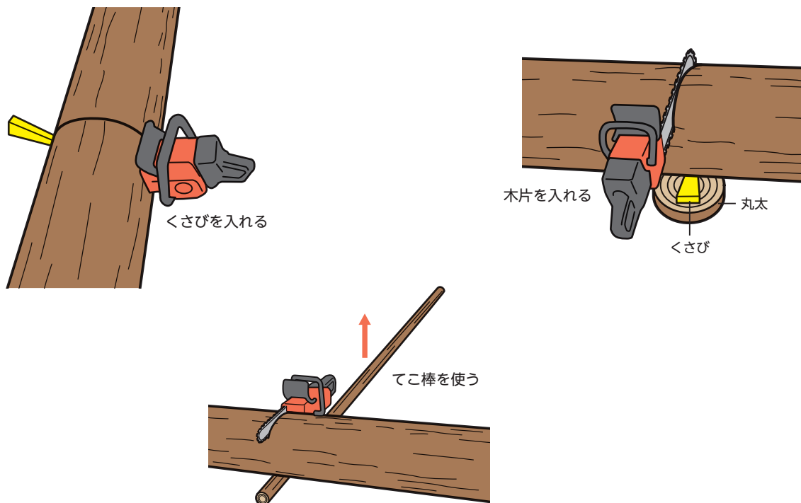
図13-14 挟まったチェーンソーの抜き方
