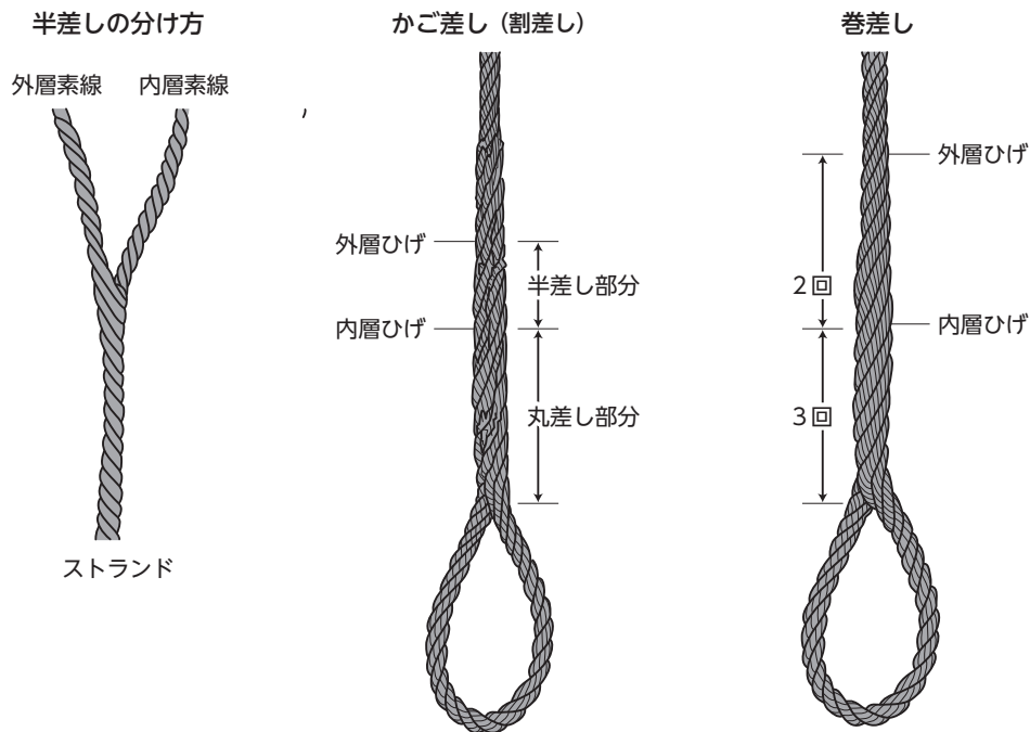
図7-12 アイスプライス加工方法—かご差し、巻差し
