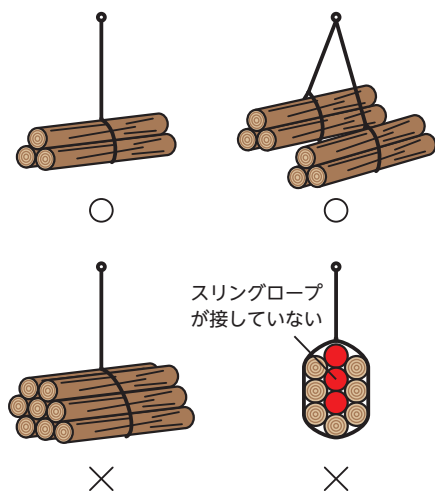
図20-14 スリングロープ1本でしぼる 吊り荷の本数は3本まで
