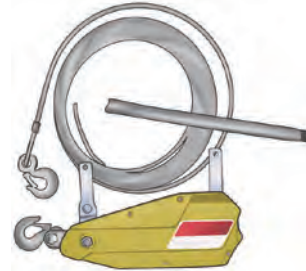
図 17-18 けん引具(チルホール)
