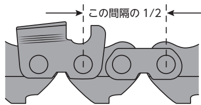
図6-10 ピッチ
