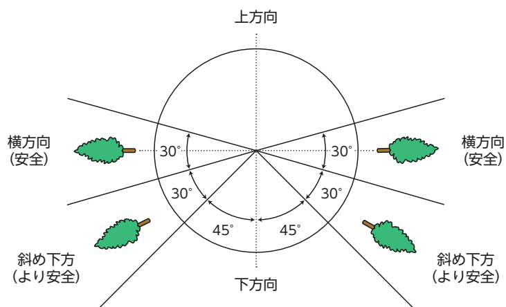
図 15-13 安全な伐倒方向
