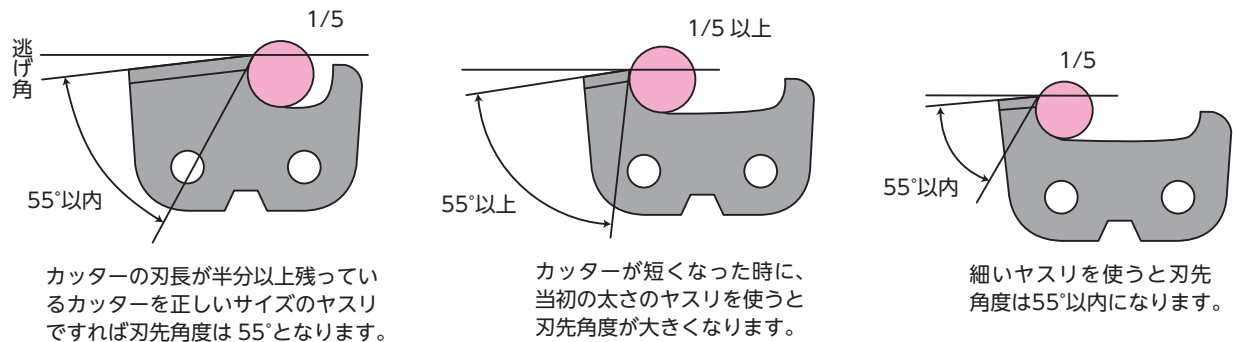
ず あしか けい 図6-20 短くなったカッターとヤスリの径
