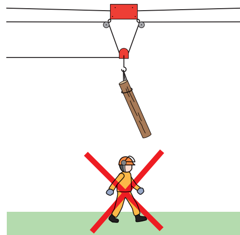
図20-15 作業者は主索の下に入らない
