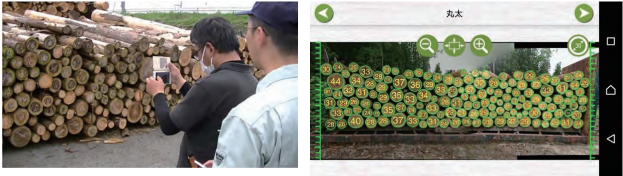
図2-12 スマホ、タブレットの撮影画像で検知できるシステム
