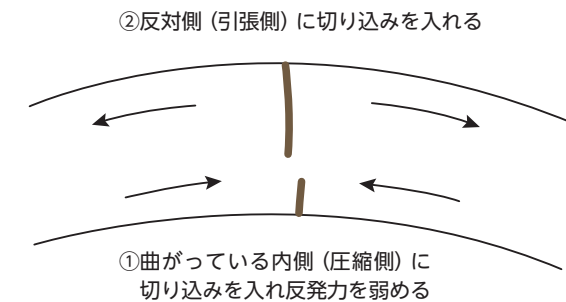
図10-16 湾曲して力が加わった木を切る手順
