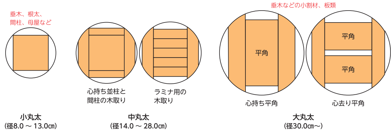
図 13-15 径級別の木取りの例
