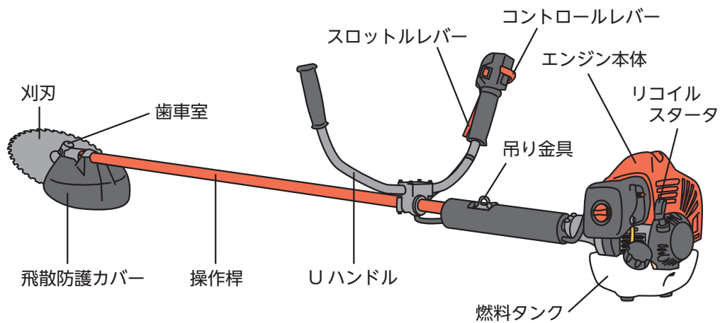
ず かりはらいき こうぞう 図10-5 刈払機(Uハンドル)の構造
