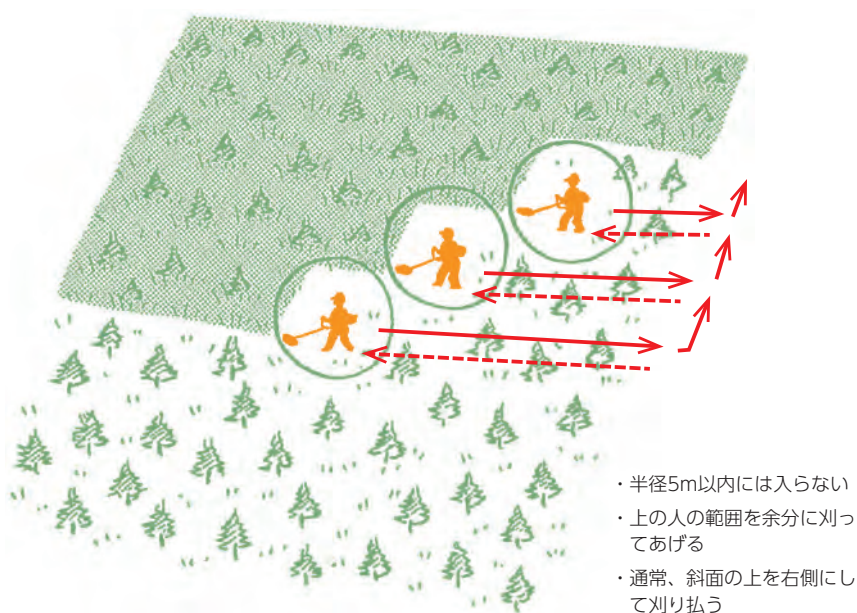
図10-9 上下作業の禁止と進行方向
