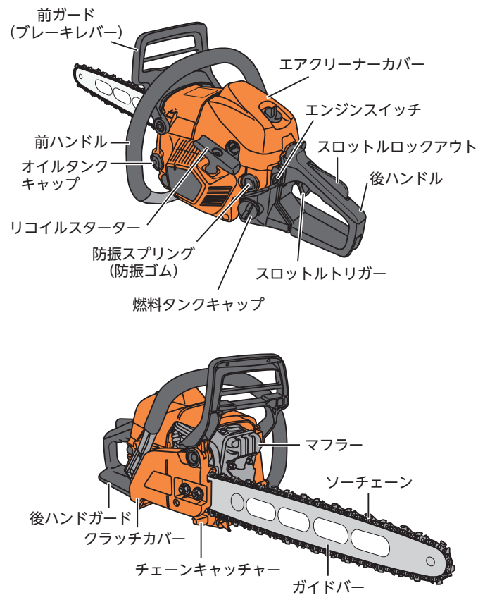
図6-1 エンジンチェーンソー（リアハンドル型）の構造と各部名称
