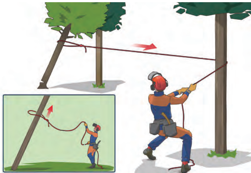
図19-11 ロープを使用したかかり木処理
