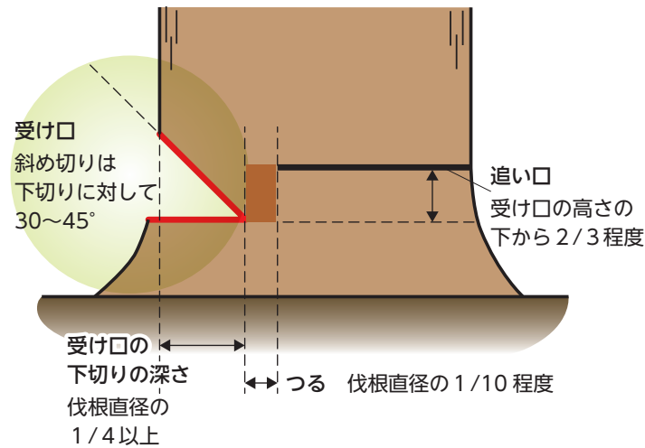
図17-9 受け口切り
