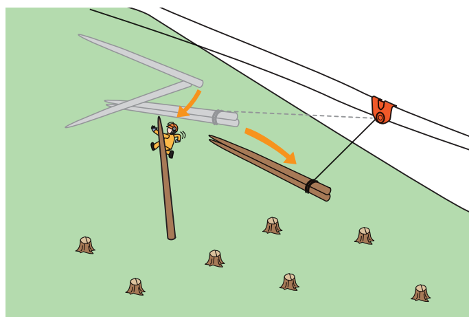
図 20-3 吊り上げた材が動き、作業者を強打 材を吊り上げたことで斜面の材が滑落し、作業者を直撃
