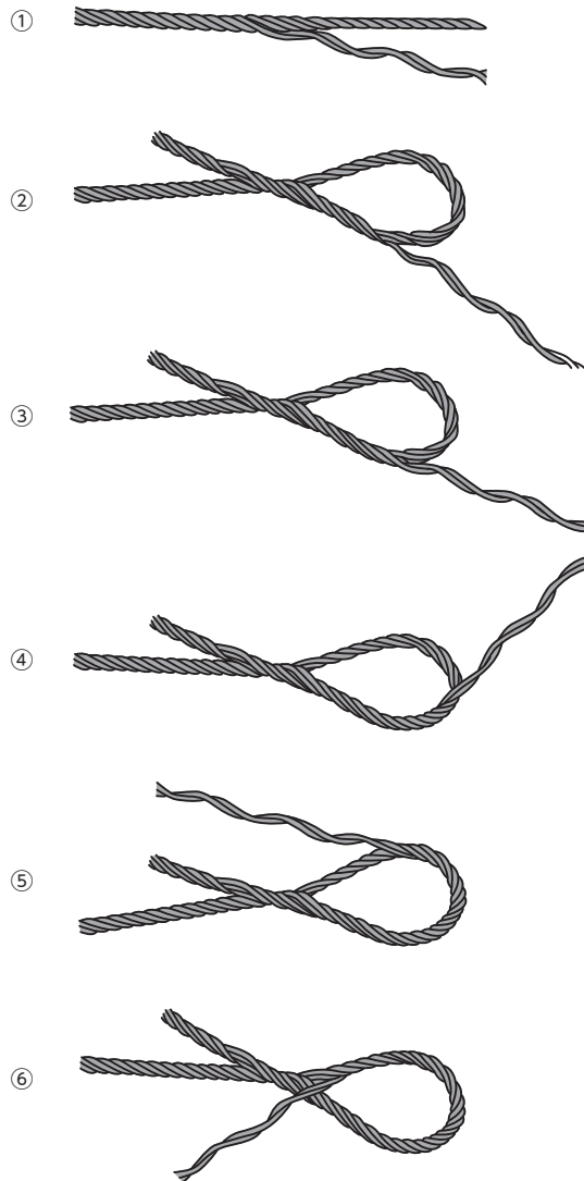
図7-13 フレミッシュアイの加工方法
