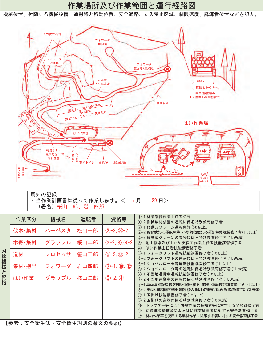
図 1-4 作業計画の記載例 (木寄せ、集材作業の計画書②) 資料：厚生労働省委託 森林環境アライズ「安全な作業に必要な作業計画の作成支援」2013/1 14 無災害の推進、チームワークとコミュニケーション、業務効率化の推進
