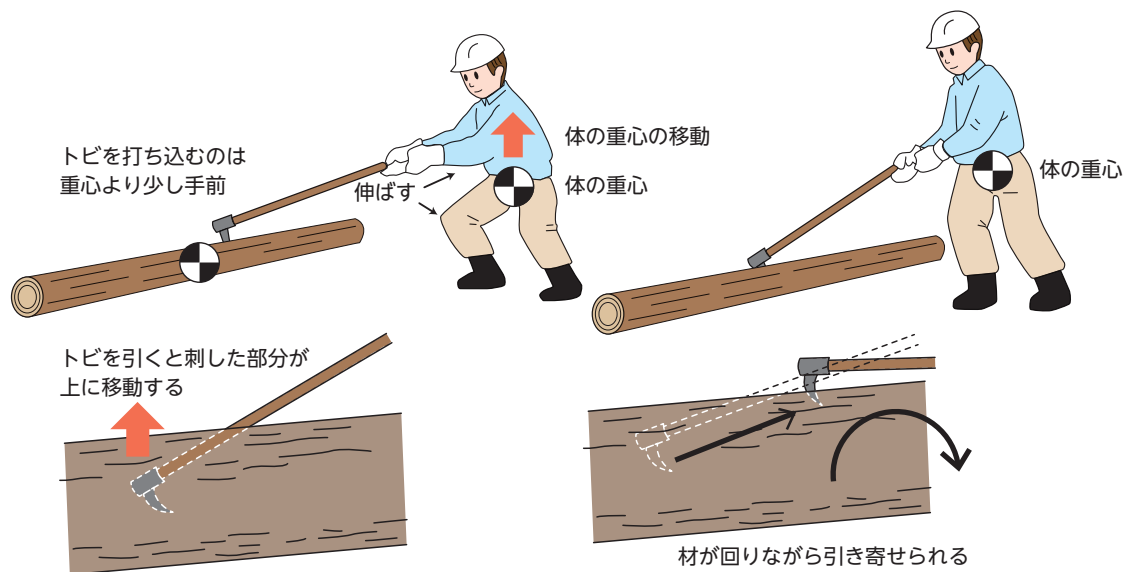
図 20-9 トビで材を回転させながら引く
