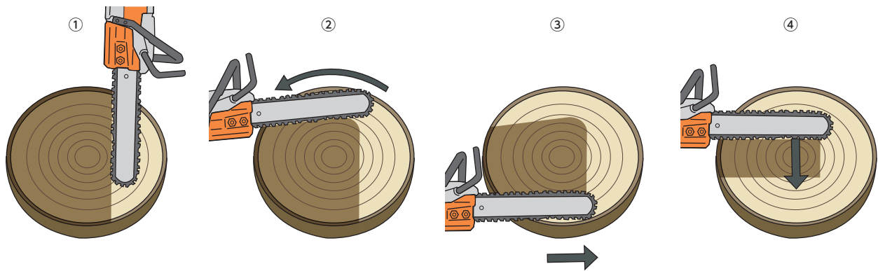
図13-9 材がガイドバーの長さよりも大きい場合(片持ち材)
