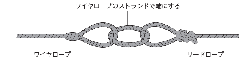
図7-15 ソワ(索輪)結び加工
