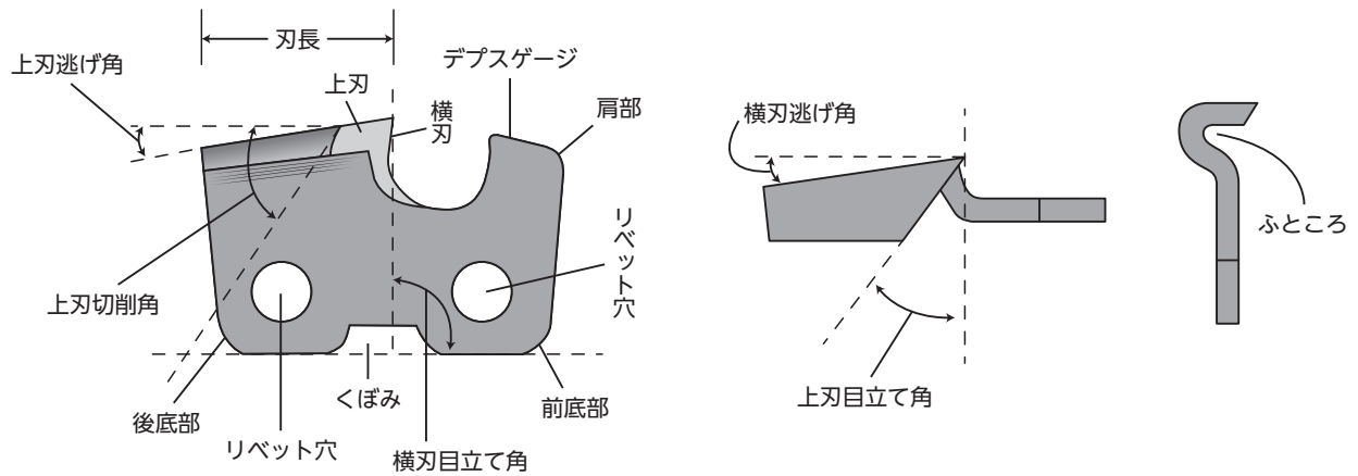
図6-5 カッター各部の名称
