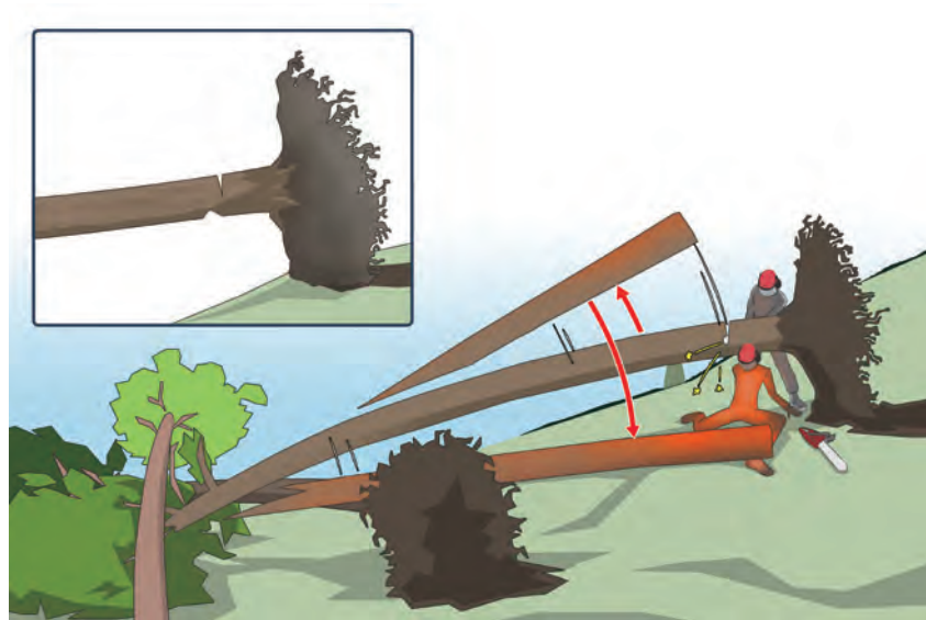
図19-22 風倒木を鋸断中、元口が跳ね返って直撃された
