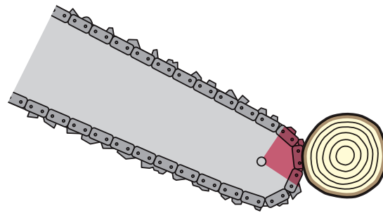
図15-11 ガイドバーの先端上部が、キックバック発生位置
