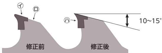
図5-14 チップソーの目立て 目立ては①から②、刃の背にかけて約10~15度の角度に軽く研磨して仕上げてください。なお、スクイ面（図①）は磨耗程度が少ないので、現状に合わせて研磨します。
