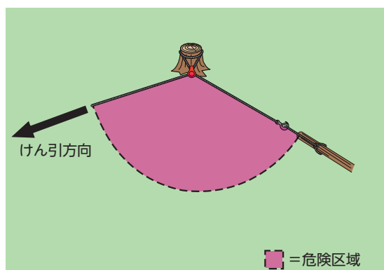
図 20-2 荷かけ作業中の内角作業はしない
