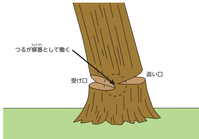
図15-17 つるが蝶番として働く つるを適切に作り、機能させます
