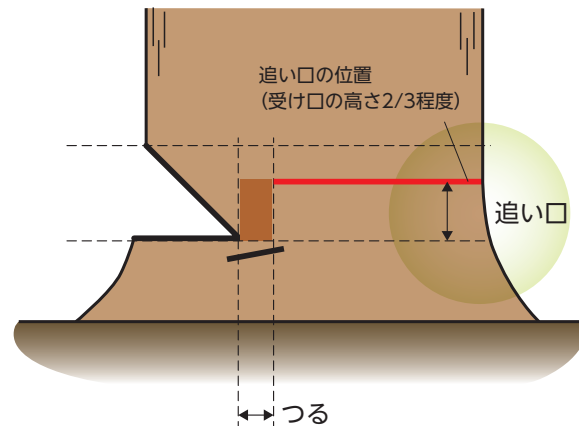
図17-13 追い口の位置
