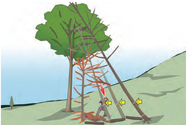
図 19-17 かかり木となっていた木を元玉切りで処理中、先端部が落下し、作業者に激突
