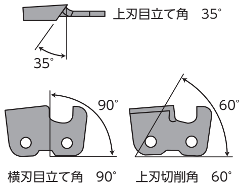
図6-13 チッパー型
