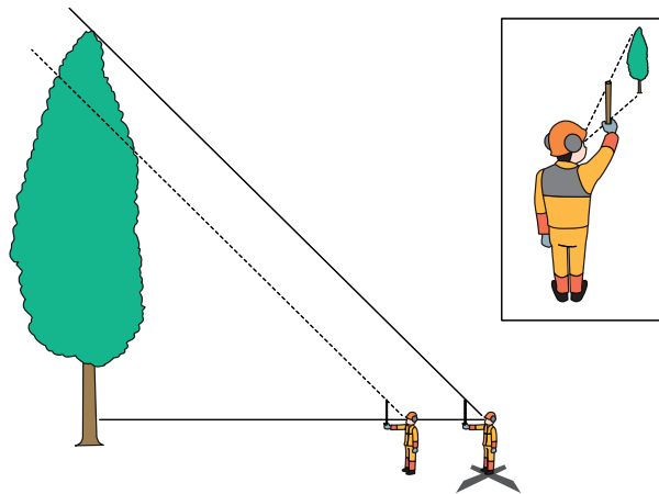
図 15-2 伐倒木を伐倒した時、その先端がどこまで来るかを測る方法
