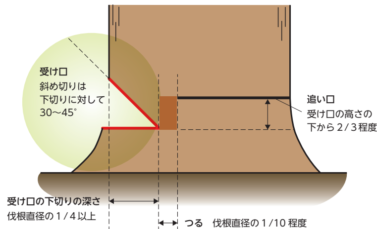
図15-15 受け口と追い口、つるの関係(横から)
