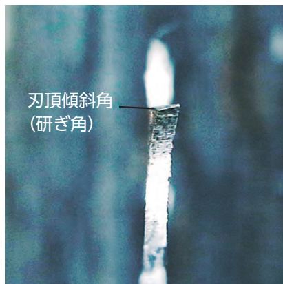
写真5-1 刃頂傾斜角
