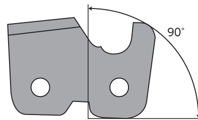
図6-23 バックスロープ型
