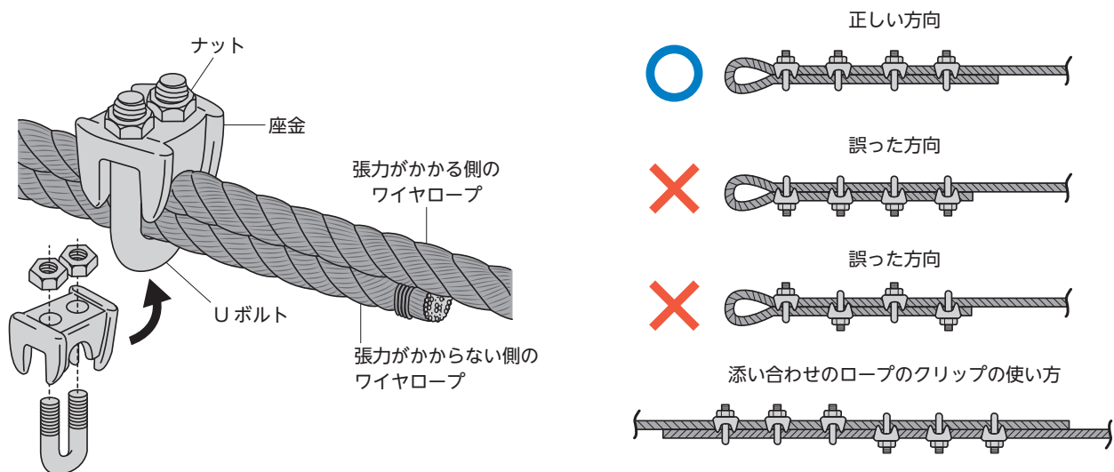
ず 図7-8 クリップの止め方 と かた
