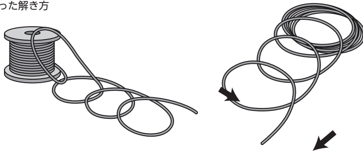
図7-3 ワイヤロープの解き方
