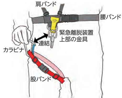
図5-5 緊急離脱装置と股バンド
