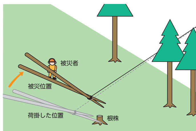
図 20-12 横取り中の材が立木に当たり旋回し、作業者に激突 木寄せ中の材が根株等にかかったことで、材が旋回し被災者を直撃した
