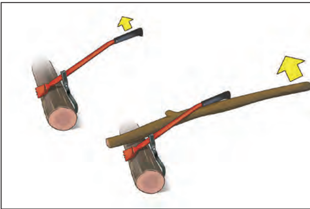
図 19-7 フェリングレバーによる木の回転。フェリングレバーと現場で調達したてこ棒を併用すると、大きな力で木回しが可能となります。
