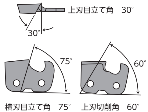
図6-14 チゼル型
