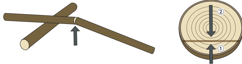
図13-8 片方の端だけで支えられている材(片持ち材)の造材
