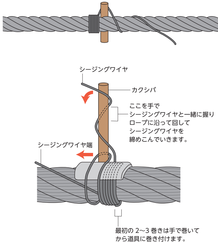
図7-7 切断箇所を針金などで巻き付けるシージングの方法
