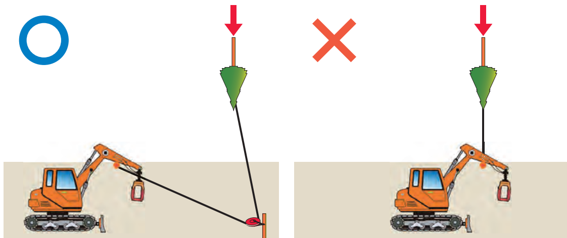
図20-4 正しい木寄せ作業と誤った木寄せ作業
