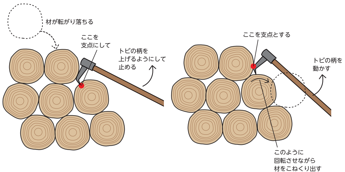
図 20-10 積み上げた材の扱い方
