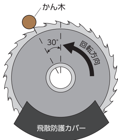
図10-13 かん木等の刈り払い位置
