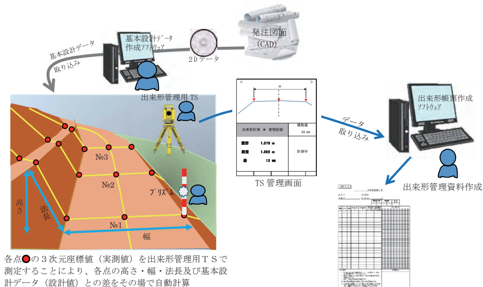
図2-8 ICTを活用した出来形管理
