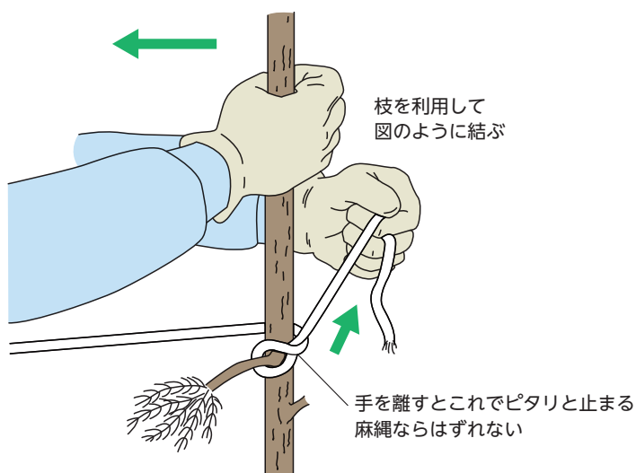
ず むす かた ゆきお 図10-18 ひもの結び方(雪起こし)
