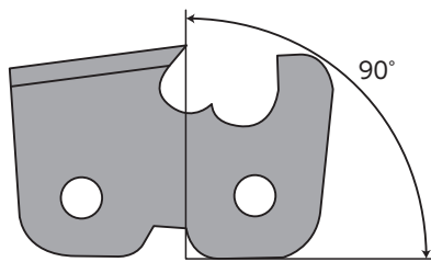
図6-22 フック型
