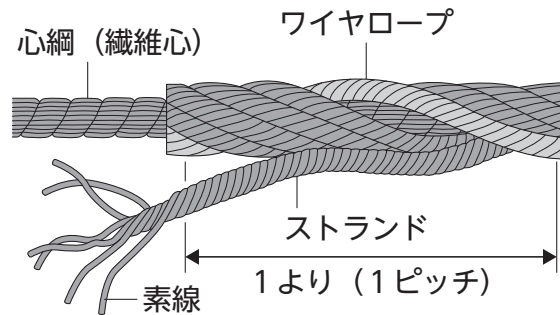
図7-1 ワイヤロープの構造
