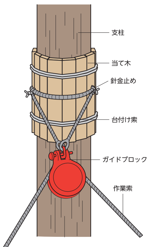
図20-6 当て木とガイドブロック等の取り付け(例)
