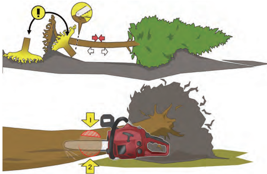
図 19-20 曲がっている木の切り離し方法 曲がりの内側（圧縮力）から切れ目を入れてから外側（引張力）から切断します。
