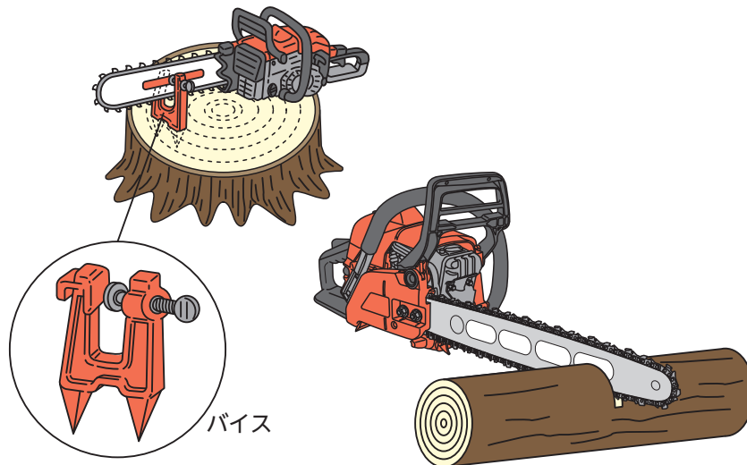
図6-12 チェーンソーの固定方法の例
