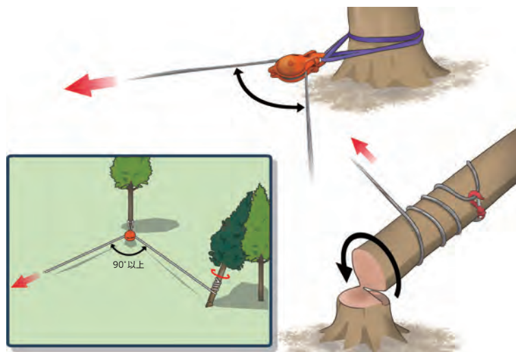
図 19-2 けん引具等を使用し、かかり木が回転するようにはずします。
