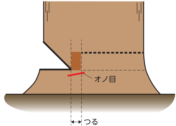
図17-11 オノ目を入れる
