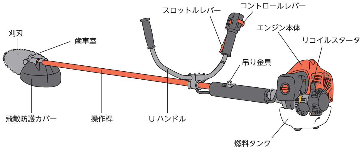
ず かたかけしきかりはらいき 図5-1 肩掛式刈払機(Uハンドル)
