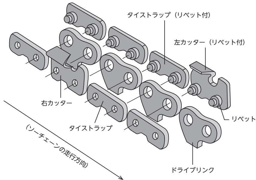
図6-4 ソーチェーンの構造と名称
