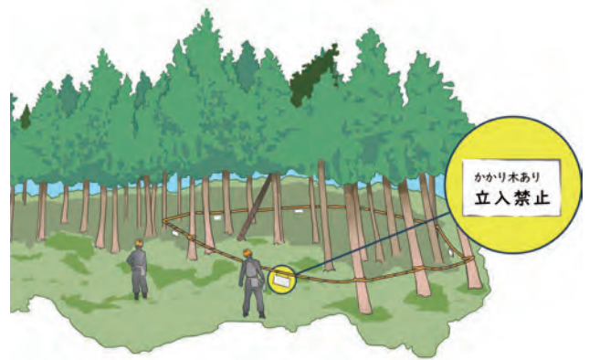
図 19-16 かかり木を一時的に放置せざるを得ない場合、縄張り等による立入禁止の措置を行う
