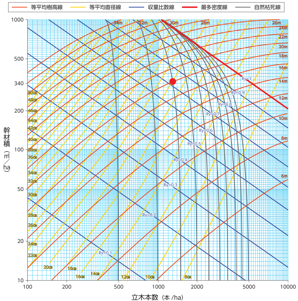
ず りんぶんみつどかんりす れい 図 14-17 林分密度管理図の例
