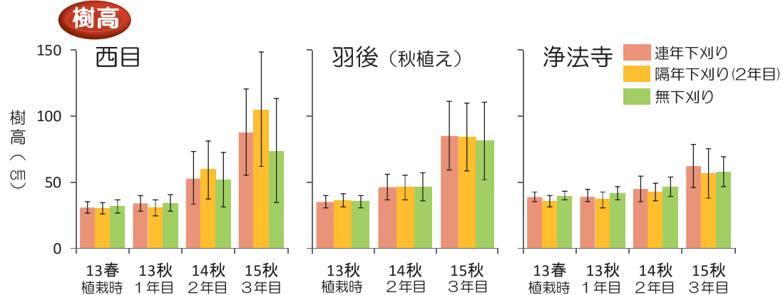
スギコンテナ苗植栽地における下刈り有無別の樹高成長
