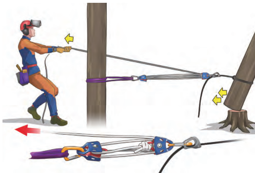
図19-12 ヒールブロックを使ったかかり木処理
