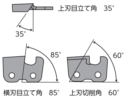
図6-15 セミチゼル型
