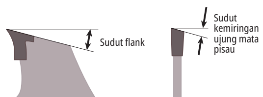
Gambar 5-15 Contoh sudut pengasahan mata gergaji bundar
