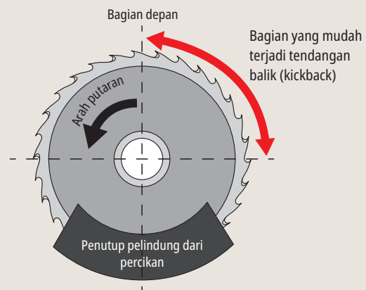
Bagian yang mudah terjadi tendangan balik (kickback)
