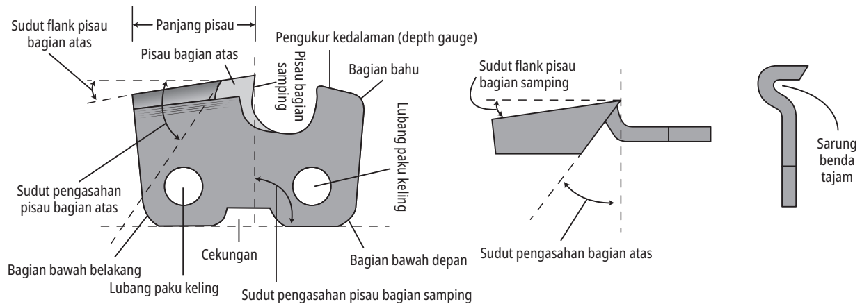
Gambar 6-5 Nama setiap bagian mata potong gergaji
