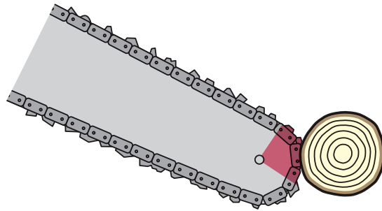
Gambar 15-11: Ujung atas bilah batang gergaji adalah titik terjadinya tendangan balik (kickback)
