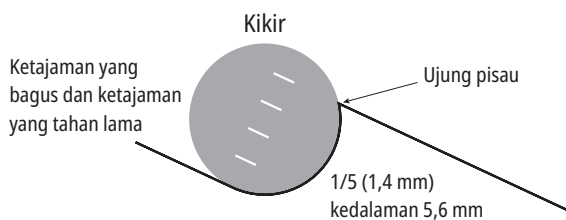
Gambar 5-11 Hubungan antara pisau pemotong rumput dan kikir bulat
