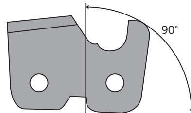
Gambar 6-23 Tipe kemiringan belakang (tipe back slope)
