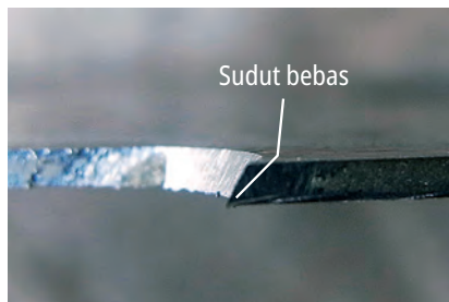
Foto 5-2 Sudut bebas
