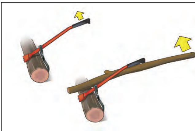
Gambar 19-7: Pemutaran kayu menggunakan tuas penebangan. Dengan mengombinasikan tuas penebangan dan batang tuas yang dibuat di lokasi kerja, pemutaran batang dapat dilakukan dengan gaya yang besar.
