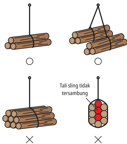
Gambar 20-14: Jumlah batang kayu yang digantung dengan satu tali sling maksimal 3 batang
