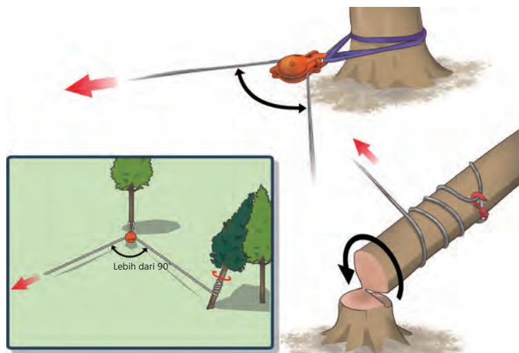
Gambar 19-2: Dengan menggunakan alat penarik/penderek, pohon yang tersangkut diputar lalu dilepaskan.
