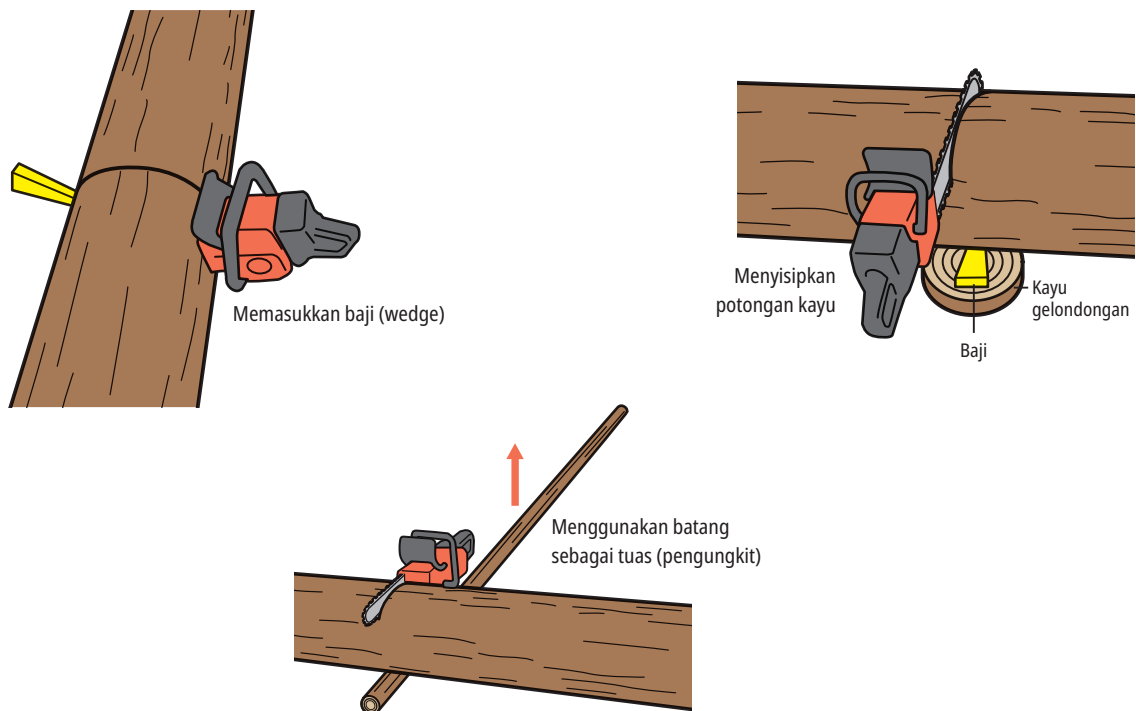
Gambar 13-14: Cara melepaskan gergaji mesin yang terjepit
