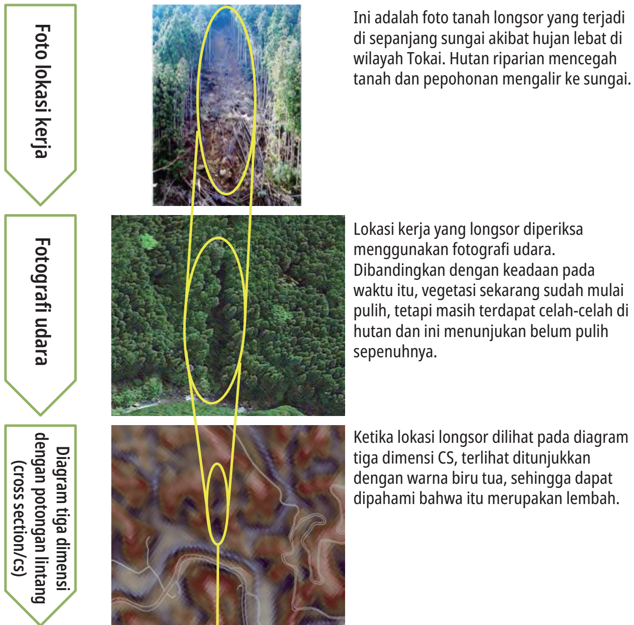
Gambar 2-3 Contoh identifikasi area berbahaya menggunakan diagram tiga dimensi dengan potongan lintang (cross section/cs) 2
