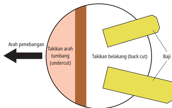
Gambar 15-18: Contoh posisi penempatan baji
