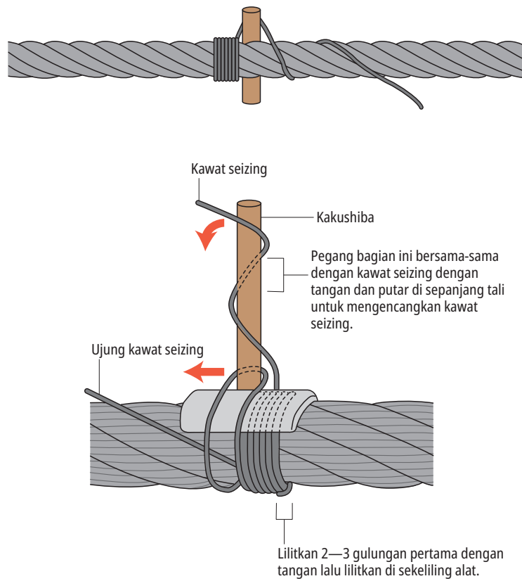
Gambar 7-7 Metode pengikat ujung tali (seizing) untuk bagian tali kawat yang dipotong dengan tali besi, dll.
