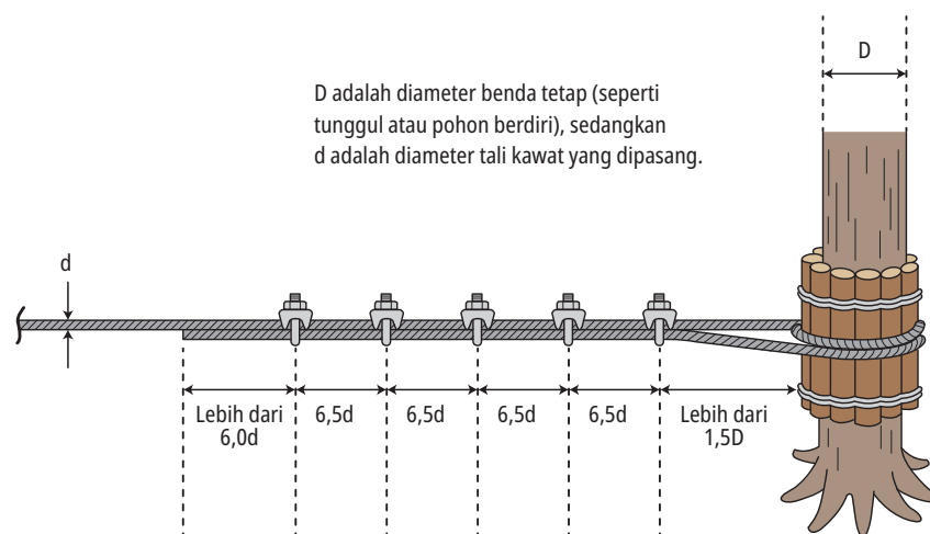
Gambar 7-9 Metode pemasangan klip (pada akar pohon, dll.)
