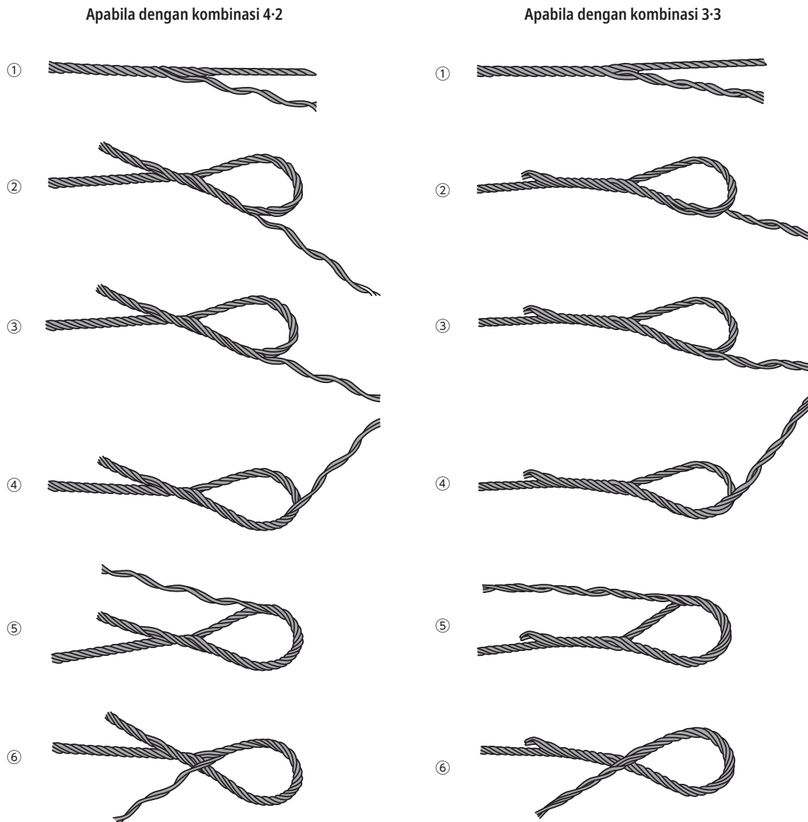
Gambar 7-13 Metode pemrosesan flemish eye
