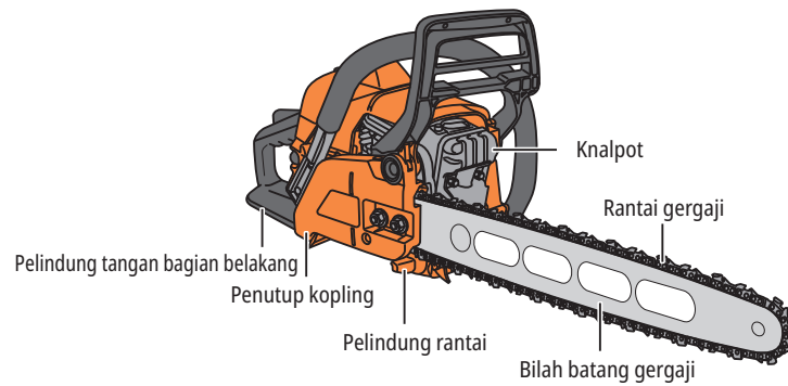
Gambar 6-1 Struktur dan nama bagian gergaji mesin (tipe pegangan belakang)
