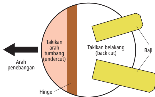
Gambar 17-14: Menggunakan baji dengan benar untuk penebangan yang aman dan pasti
