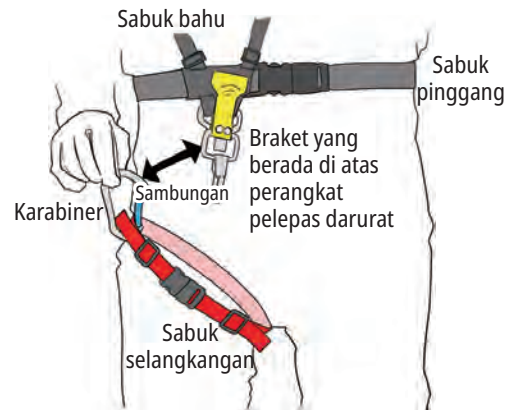
Gambar 5-5 Perangkat pelepasan darurat dan sabuk selangkangan
