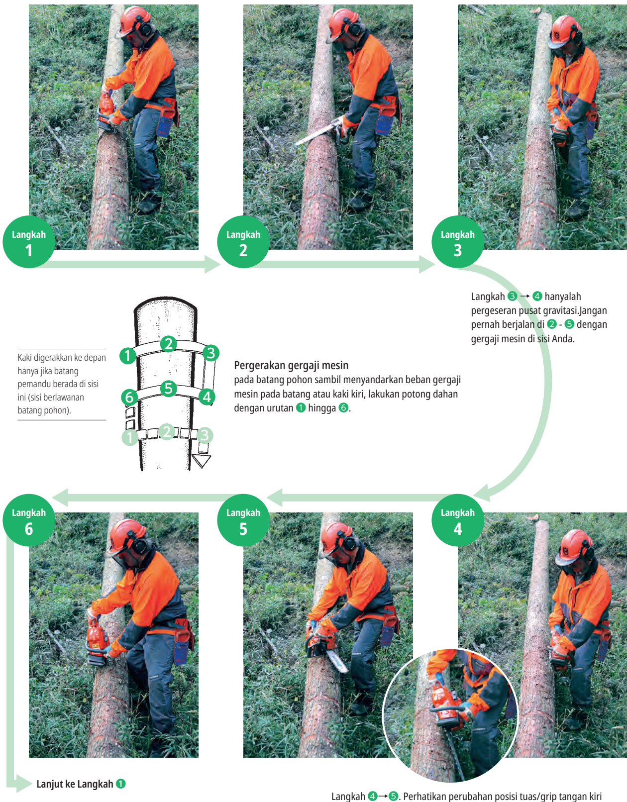
Gambar 13-6: Sistem 6 poin dilihat dari depan
