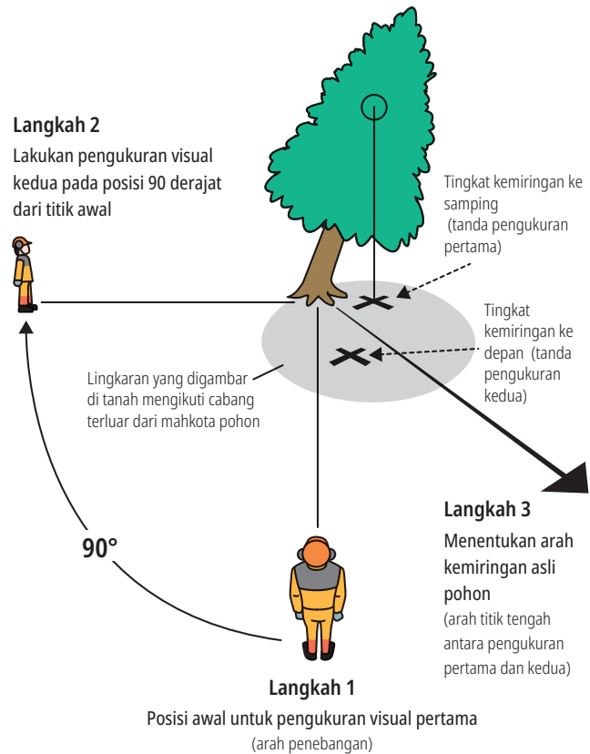
Gambar 17-2: Mengukur kemiringan pohon
