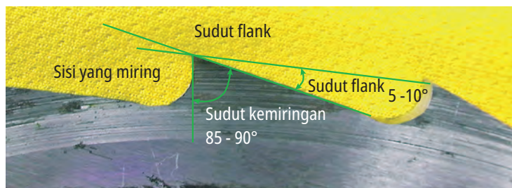
Foto 5-3 sudut kemiringan
