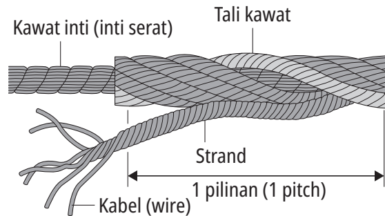
Gambar 7-1 Struktur tali kawat
