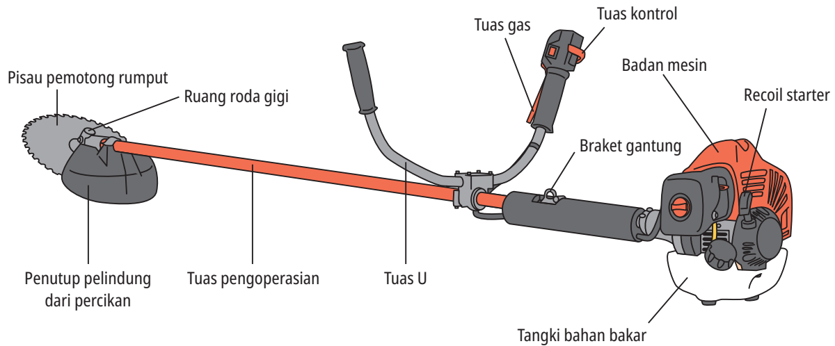
Gambar 5-1 Mesin pemotong rumput tipe bahu (tuas U)
