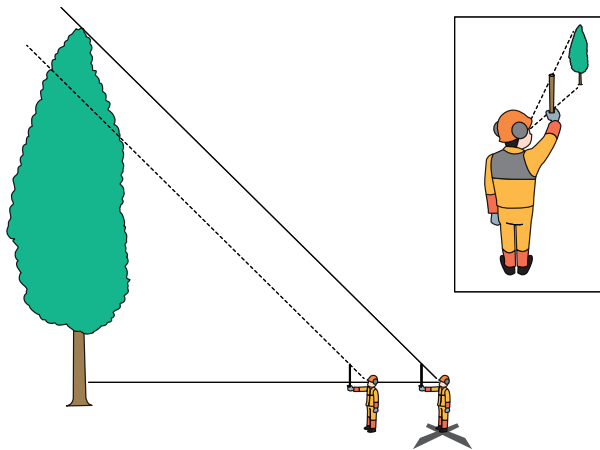
Gambar 15-2: Cara mengukur sejauh mana ujung pohon yang ditebang akan jatuh
