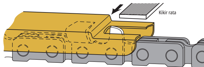
Gambar 6-24 Pengukur kedalaman (depth gauge) dan penggaris
