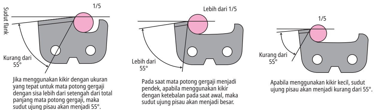
Gambar 6-20 Mata potong gergaji yang menjadi pendek dan ukuran kikir
