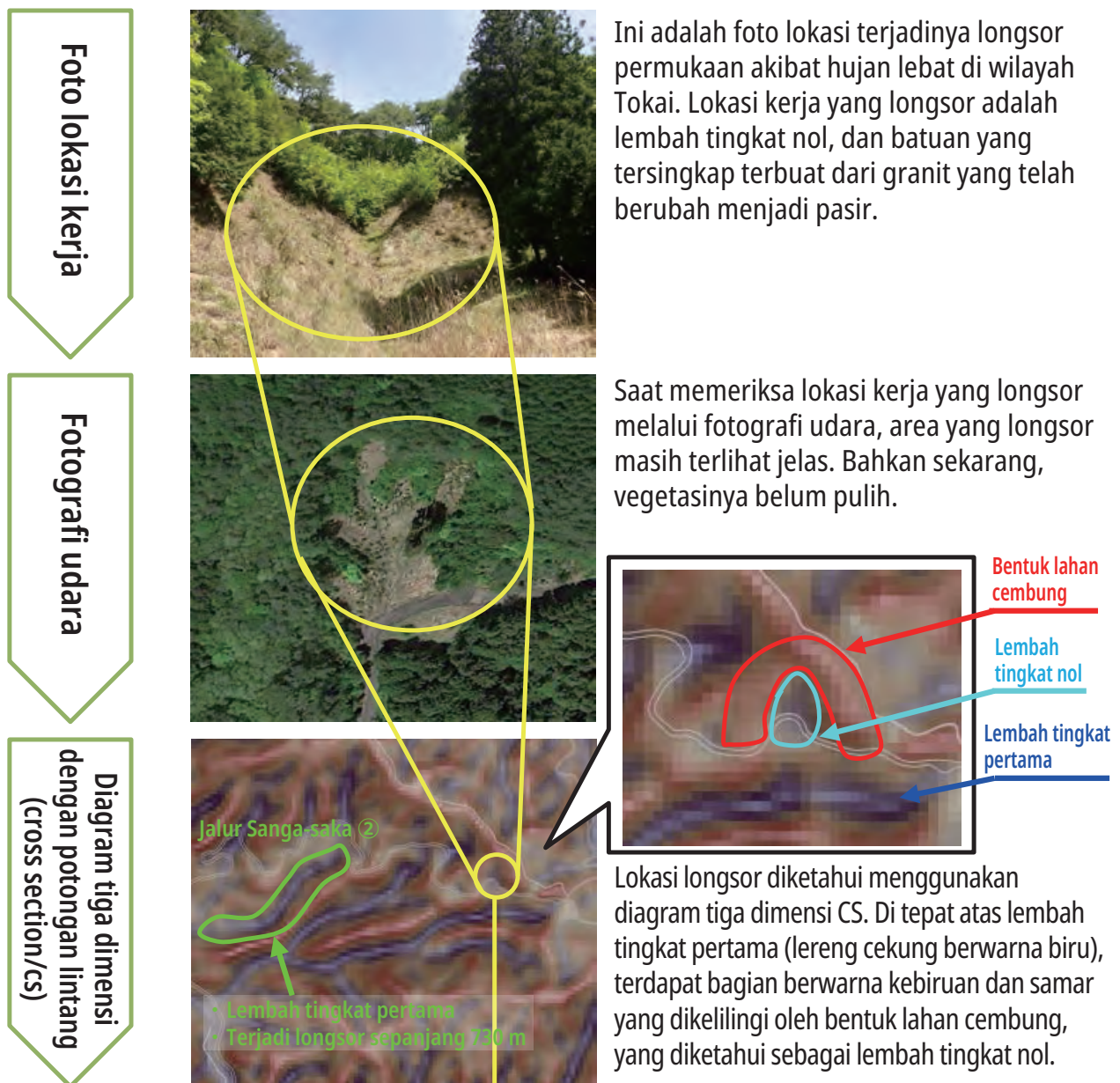
Gambar 2-2 Contoh identifikasi area berbahaya menggunakan diagram tiga dimensi dengan potongan lintang (cross section/cs) 1
