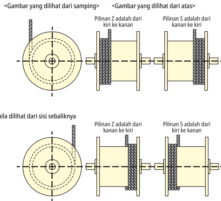
Gambar 7-5 Cara menggulung tali kawat pada drum winch mesin pengumpul kayu
