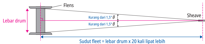
Gambar 7-6 Memasang sheave (katrol) pada jarak lebih dari 20 kali lebar drum—Sudut fleet
