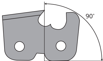
Gambar 6-22 Tipe kait
