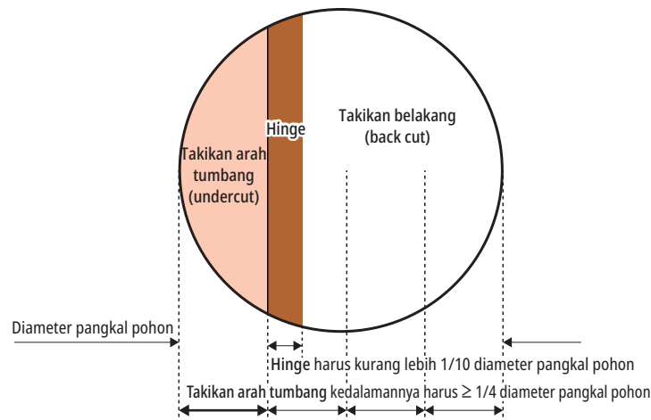
Gambar 15-16: Hubungan antara takikan arah tumbang (undercut) dan takikan belakang (back cut) serta hinge (dilihat dari atas)
