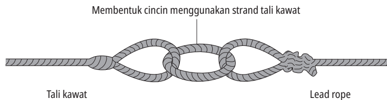
Gambar 7-15 Pemrosesan simpul lingkaran sederhana
