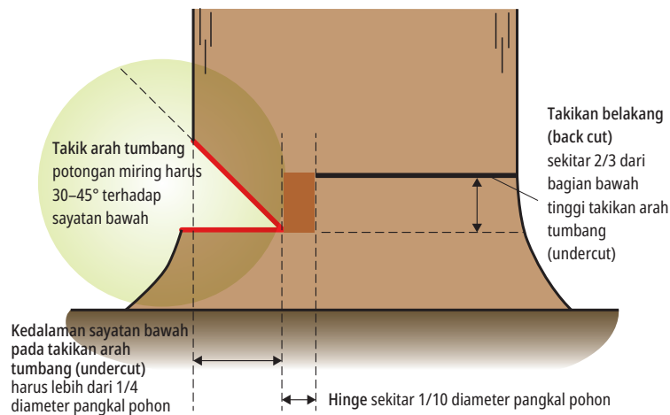
Gambar 15-15: Hubungan antara takikan arah tumbang (undercut) dan takikan belakang (back cut) serta hinge (dilihat dari samping)
