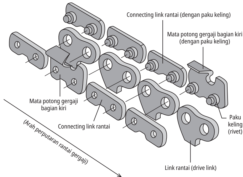
Gambar 6-4 Struktur dan nama rantai gergaji
