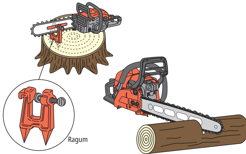
Gambar 6-12 Contoh cara mengunci gergaji mesin
