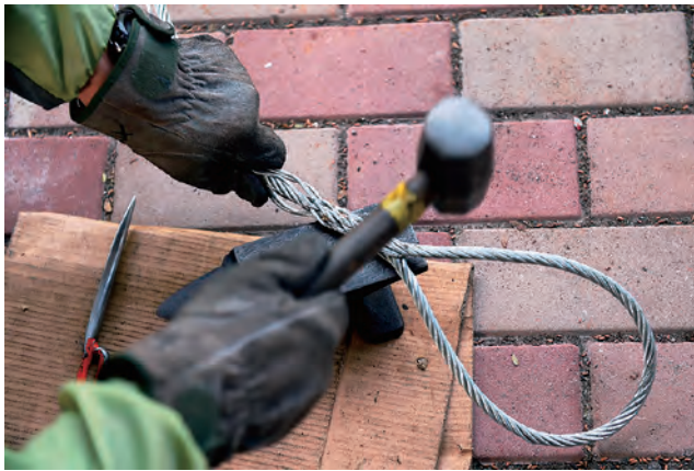
Foto 7-2 Pemrosesan eye splice
