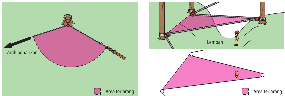
Gambar 20-2: Hindari bekerja di sudut bagian dalam saat memasang beban
