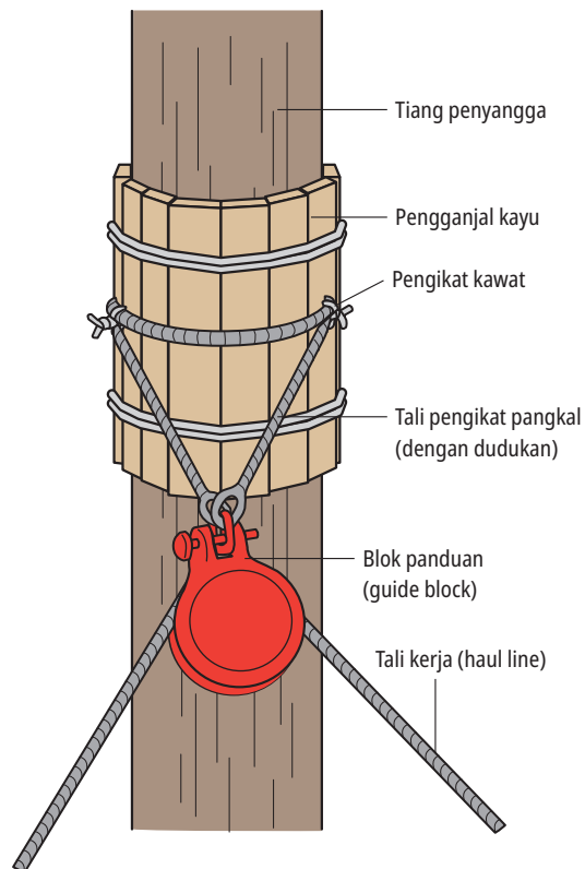
Gambar 20-6: Contoh pemasangan kayu pelindung dan guide block
