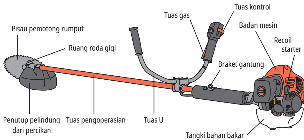
Gambar 10-5 Struktur mesin pemotong rumput (tuas U)
