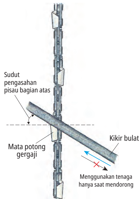
Gambar 6-19 Cara menggunakan kikir bulat
