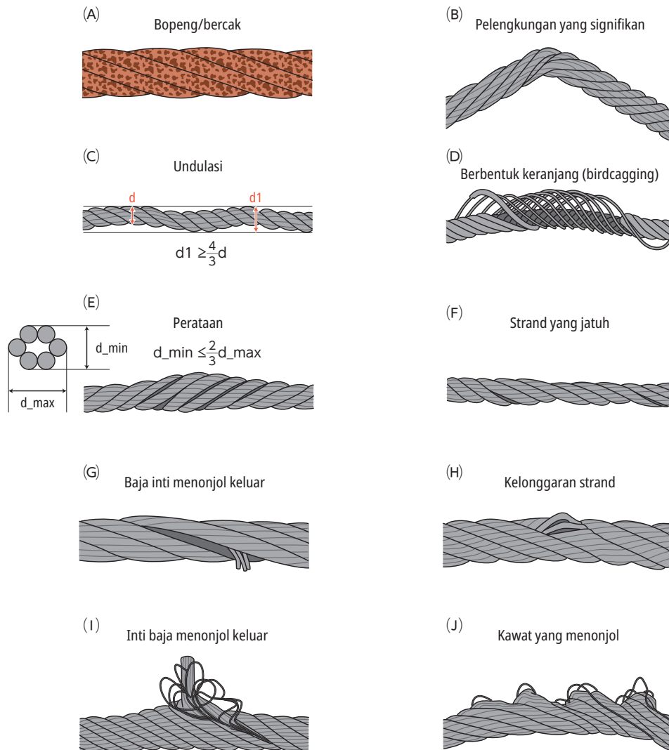
Gambar 7-10 Kriteria pembuangan tali kawat
