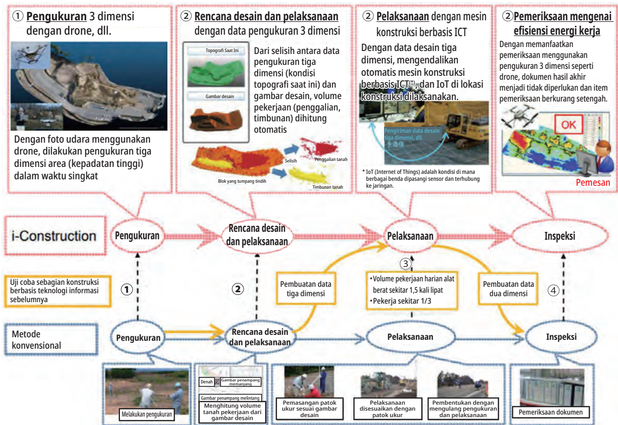
Gambar 2-1 Contoh pekerjaan tanah berbasis ICT dalam i-Construction
