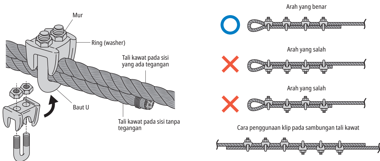
Gambar 7-8 Cara memasang klip
