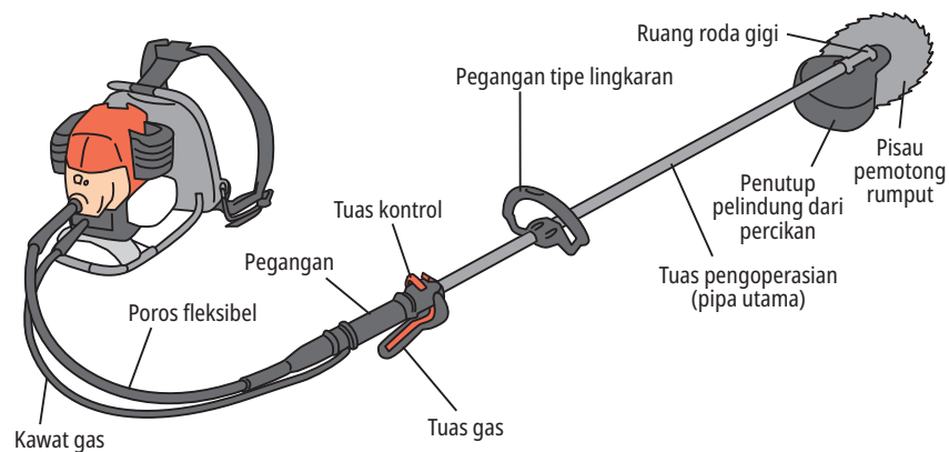
Gambar 5-2 Mesin pemotong rumput tipe ransel
