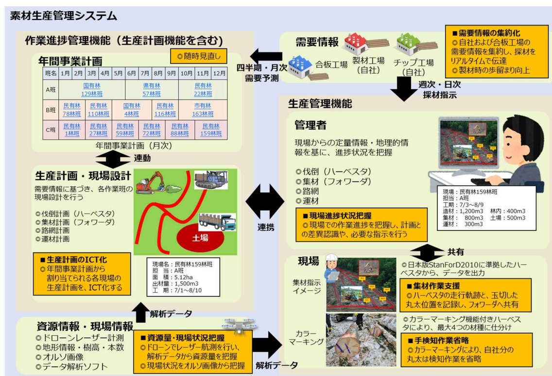
図 5 素材生産管理システム概要
