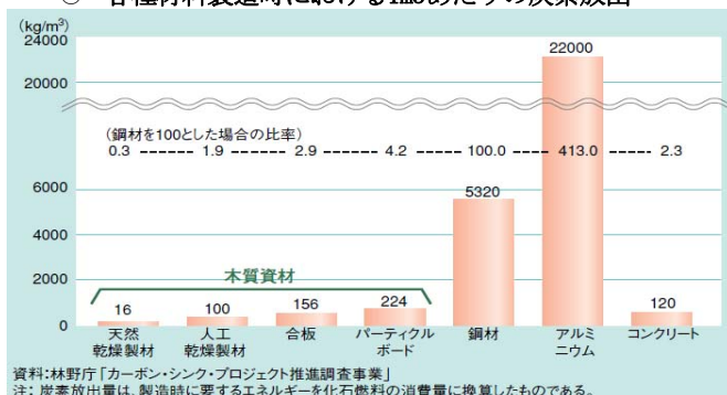
○ 各種材料製造時における1m 3 あたりの炭素放出
