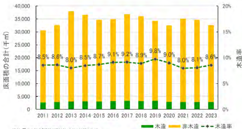
図2 着工した非住宅建築物の構造別の床面積と木造率の推移
