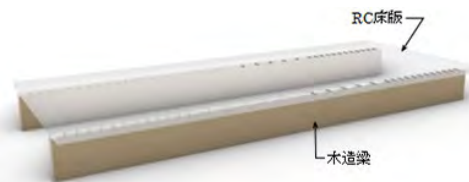
木質梁とRC床版を接合した 「合成梁構法」 *株式会社日建設計と共同開発
