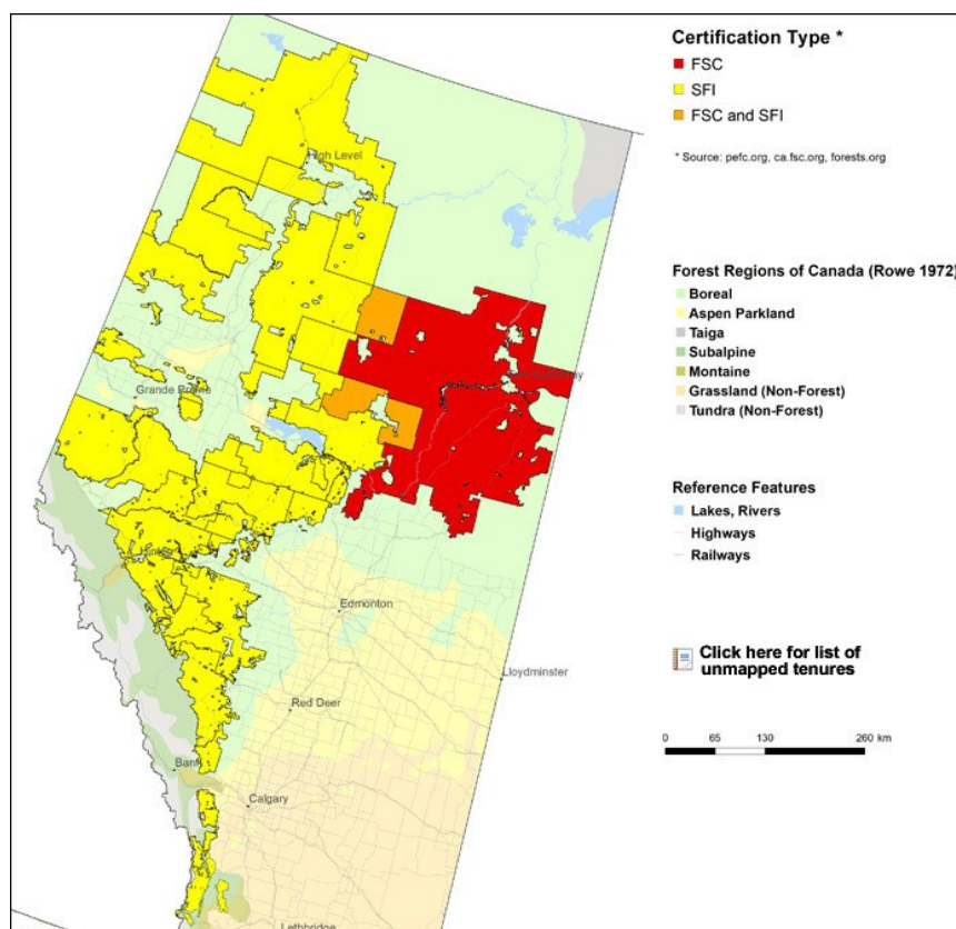
図 3-4 アルバータ州における森林認証取得エリアを示した地図 192
