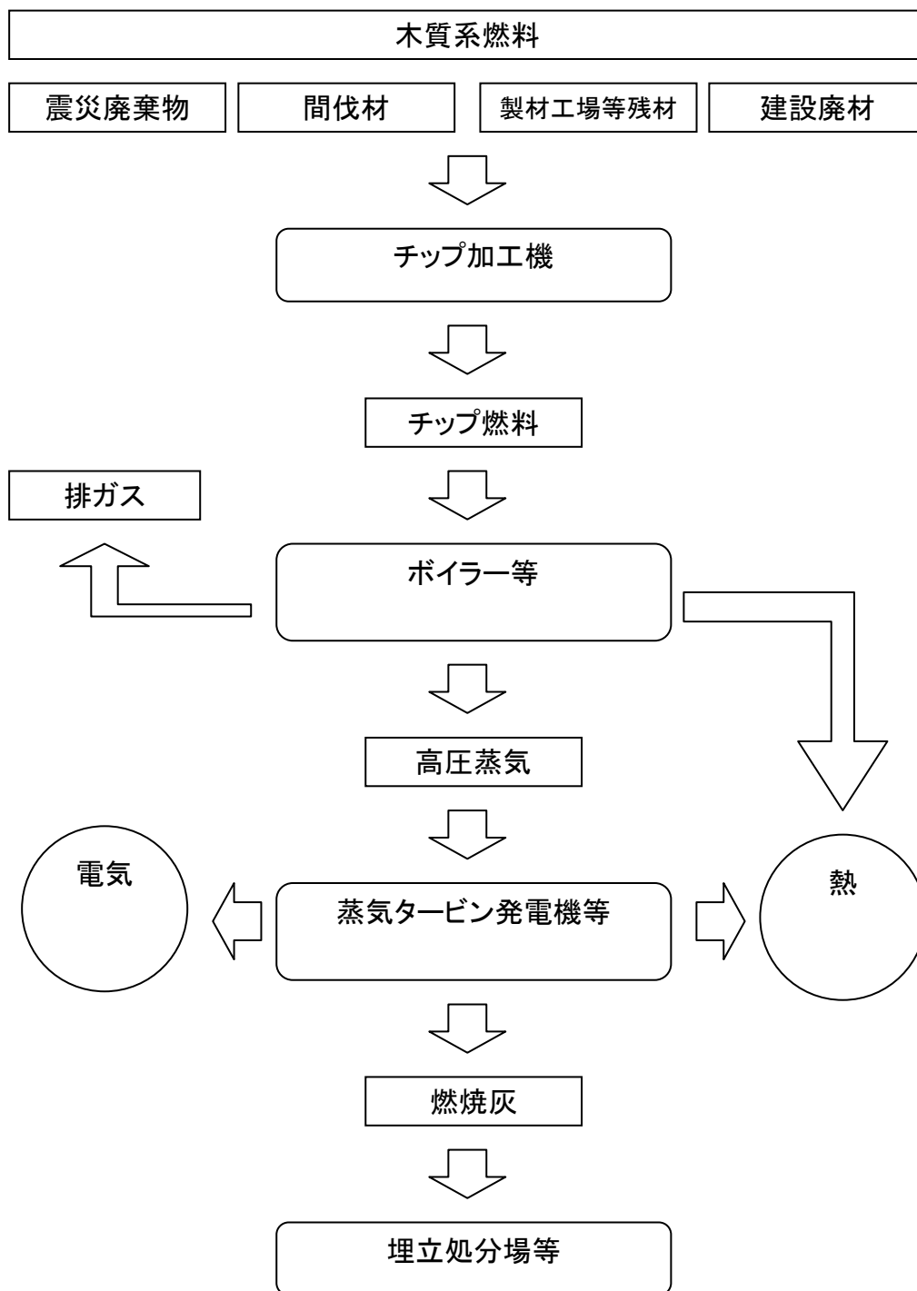
図11 木質バイオマスを利用した熱・電併給システムの概要
