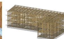
木造建築物のBIMモデル
