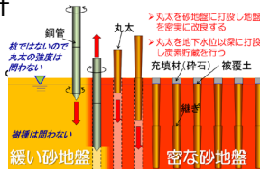
工法の原理
