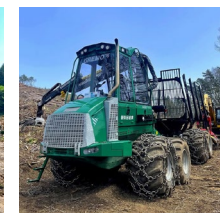
次世代型フォワーダ
