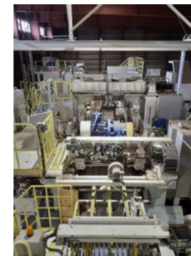
小径木用ロータリーレース
