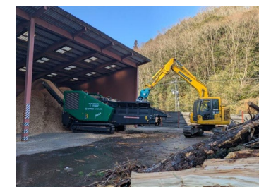
移動式チップパー(アクスター6210)
