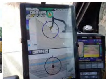
治山事業におけるICT活用事例 （MG（マシンガイダンス）付きバックホーによる掘削）
