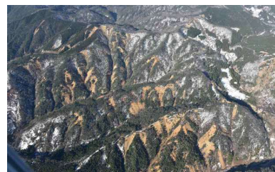
能登半島地震で発生した多数の山腹崩壊
