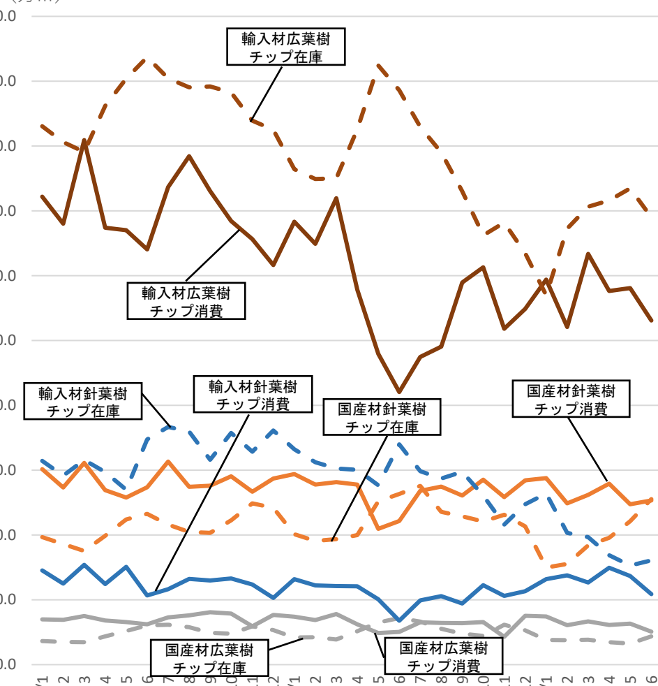
(万m 3 ) パルプ用チップの消費量・在庫量
