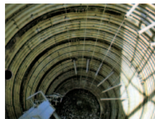
集水井工により地下水を排除
