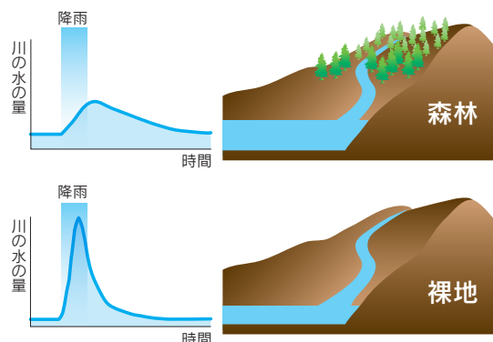
図③ 森林と裸地における斜面の降雨流出過程
