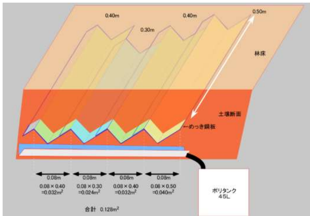
図 4-28 ゼロテンションライシメータ構造図
