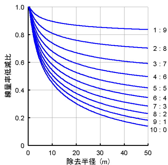
図8 空間線量率の変化に対する上下の放射性物質の比率の影響
