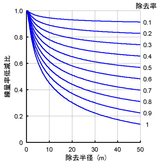
図6 空間線量率の変化に対する除去率の影響
