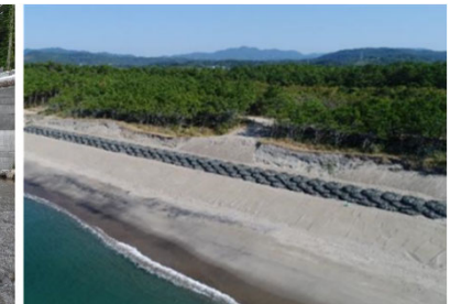
防潮工
