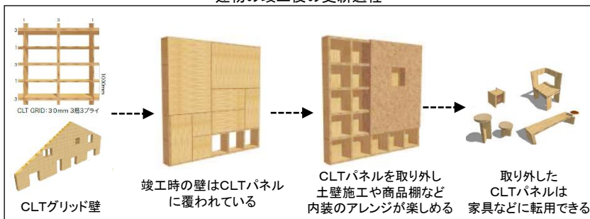
建物の竣工後の更新過程
