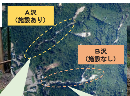
長野県下伊那郡天龍村 令和5年梅雨前線豪雨において、 流木止工が流木等を捕捉
