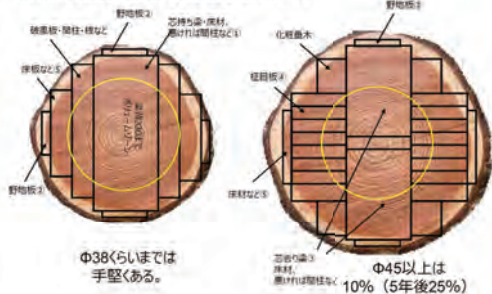
製材木取の凡例（現在とこれから）
