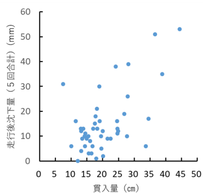
図－６ 貫入試験結果と沈下量の関係
