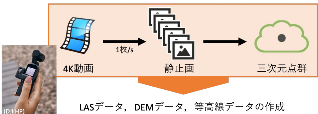
図-3 Osmo pocket を使った動画撮影と SfM 処理のフロー
