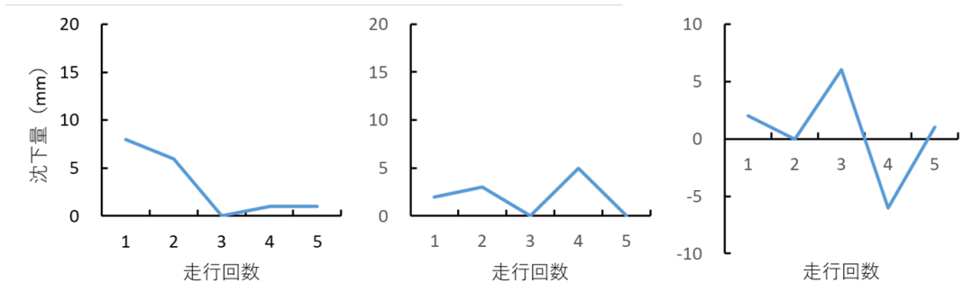
図－４ 走行回数と路面沈下量の関係
