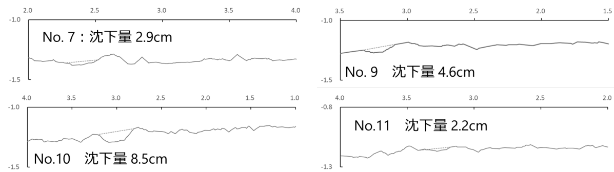
図ー3 SfMによる点群から作成した測線部の横断面図 横軸は水平距離、縦軸は垂直距離を表す（単位：m）。走行前の推測路面を点線で示し、 この推測路面から求めた沈下量を図中に記す。
