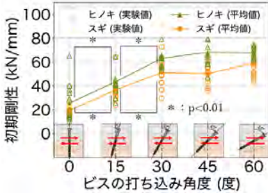
図2：CLTとコンクリートを接合するビスの打ち込み角度と初期剛性の関係
