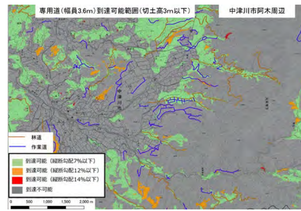
図 3：路網計画地選定支援図
