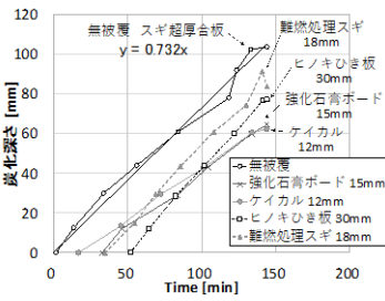
図4：スギ超厚合板の被覆仕様ごとの炭化深さ
