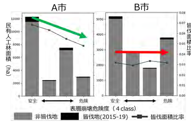
図 2：表層崩壊危険度と皆伐面積比率の関係
