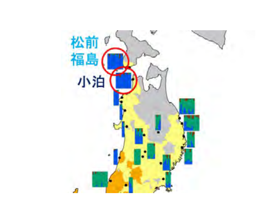
図 1：カシノナガキクイムシ集団解析結果 北海道南端の集団が対岸の青森県津軽半島集団と遺伝的にほぼ同一であることを示す。
