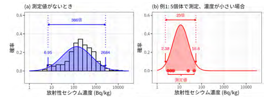
図1：当年枝の放射性セシウム濃度の予測の例 40調査区（20～40m四方）で418個体の当年枝の放射性セシウム濃度を統計モデルにより解析し、 調査区ごとに平均は異なるが標準偏差は一定 であることを解明
