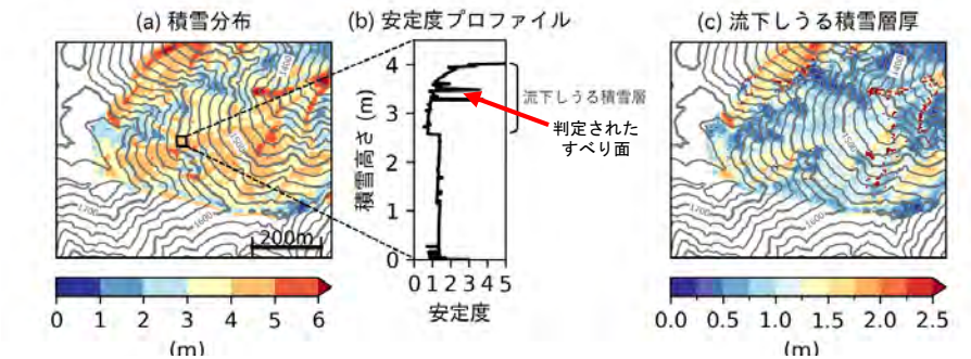
図2：雪崩発生時の積雪量（a）、積雪内での安定度プロファイル（b） 流下しうる積雪層厚（c）の推定図
