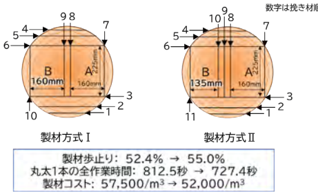
図1：効率的製材方法の提案
