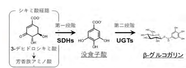
図1 草本モデル植物による加水分解性タンニンの生合成経路の再現 ユーカリにアルミニウム耐性をもたらす加水分解性タンニンの生合成経路の中間代謝物である没食子酸とβ-グルコガリンの生成を草本モデル植物で再現することに成功した。
