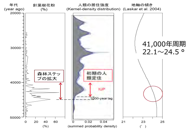
図 3：針葉樹花粉の割合と人類の居住強度の比較 針葉樹を主とする森林ステップの拡大と初期の人類定住がほぼ同時期に起きていることを示している
