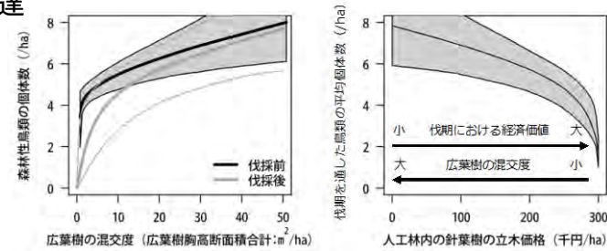
図2 広葉樹の量（左）と山元立木価格（右）に対する森林性鳥類個体数の反応 伐採前後の広葉樹の胸高断面積合計と森林性鳥類の個体数の関係（左）から、山元立木価格と伐期を通した平均個体数の関係（右）を導いた。生物多様性保全上望ましいと考えられた広葉樹50本保持/haは、広葉樹胸高断面積合計の3.2 m²/haに相当する。
