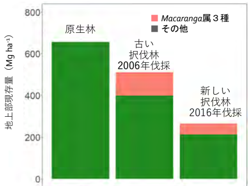
図 1：マレーシア・サバ州の熱帯雨林の択伐林と原生林の地上部現存量 択伐年が古いほど地上部現存量は原生林に近づく
