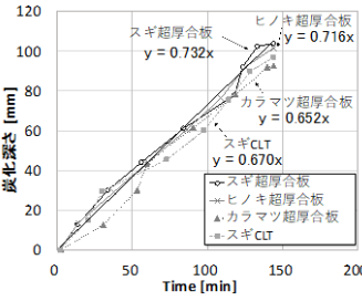
図3：無被覆試験体の炭化深さ推移
