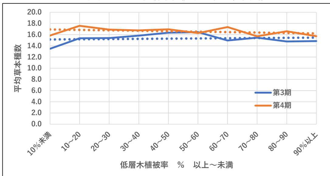
図表3-80 低層木植被率別平均草本種数
