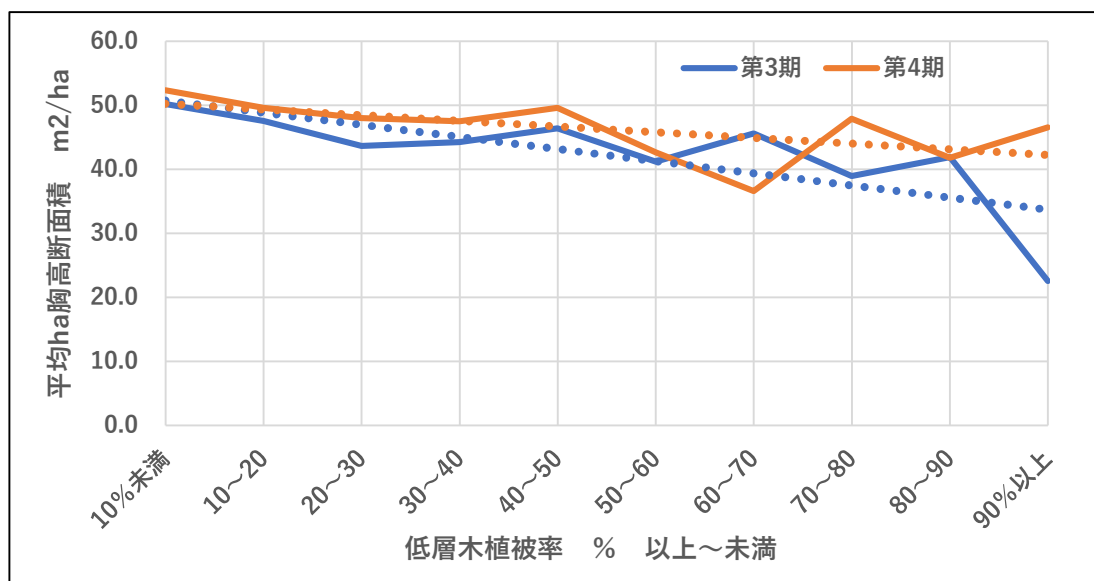
図表3-109 低層木植被率別の平均 ha 当り胸高断面積
