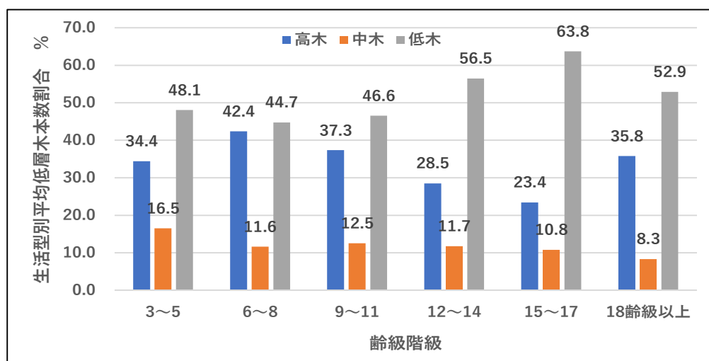
図表5-13 生活型別低層木の立木本数割合(%)
