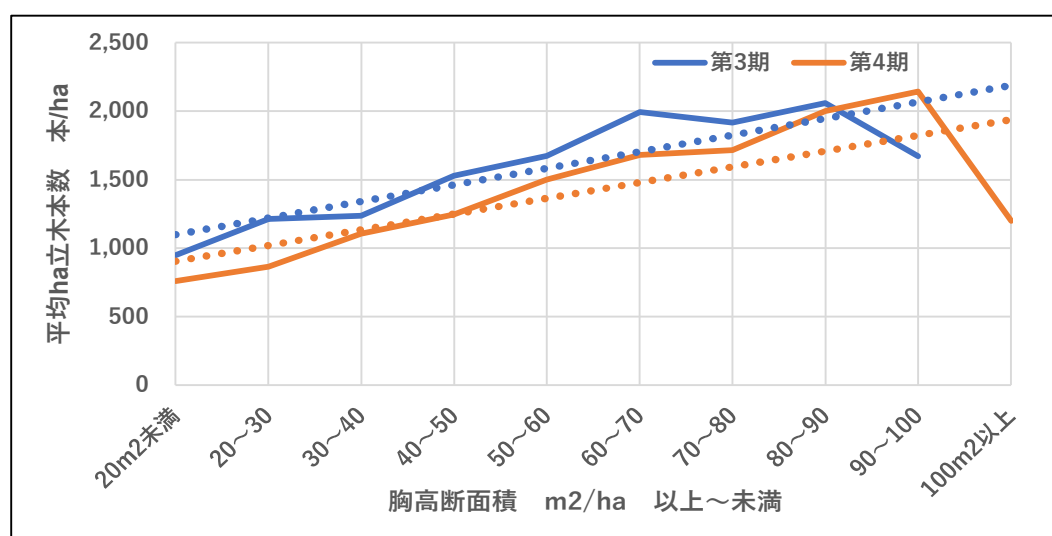
図表3-101 胸高断面積別の ha 当り平均立木本数
