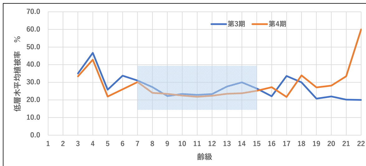
図表 5-2 齢級別の平均低層木植被率
