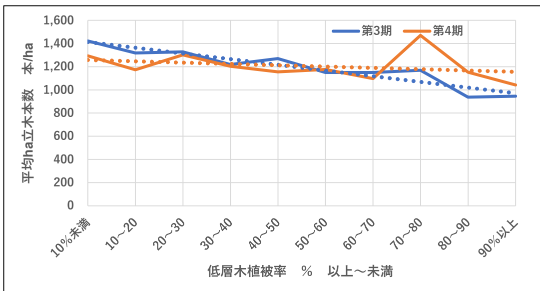
図表3-74 低層木植被率別平均 ha 立木本数
