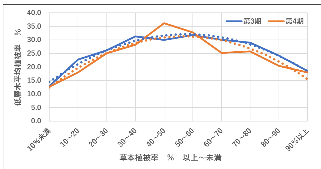
図表3-87 草本植被率別低層木平均植被率
