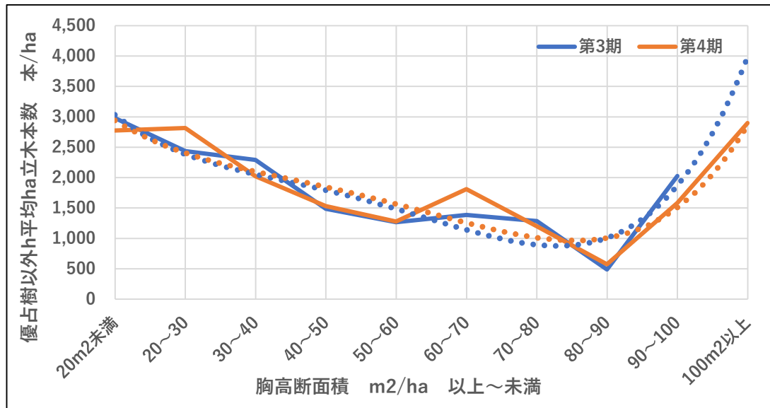
図表3-102 胸高断面積別の平均低層木立木本数
