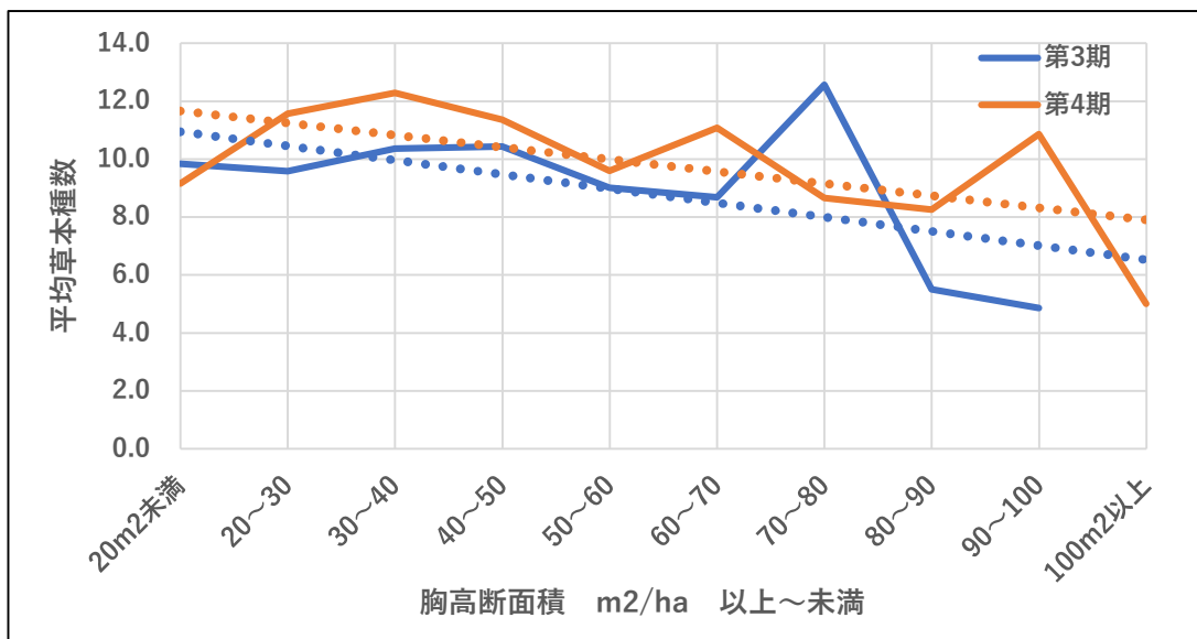
図表3-106 胸高断面積別の平均草本種数
