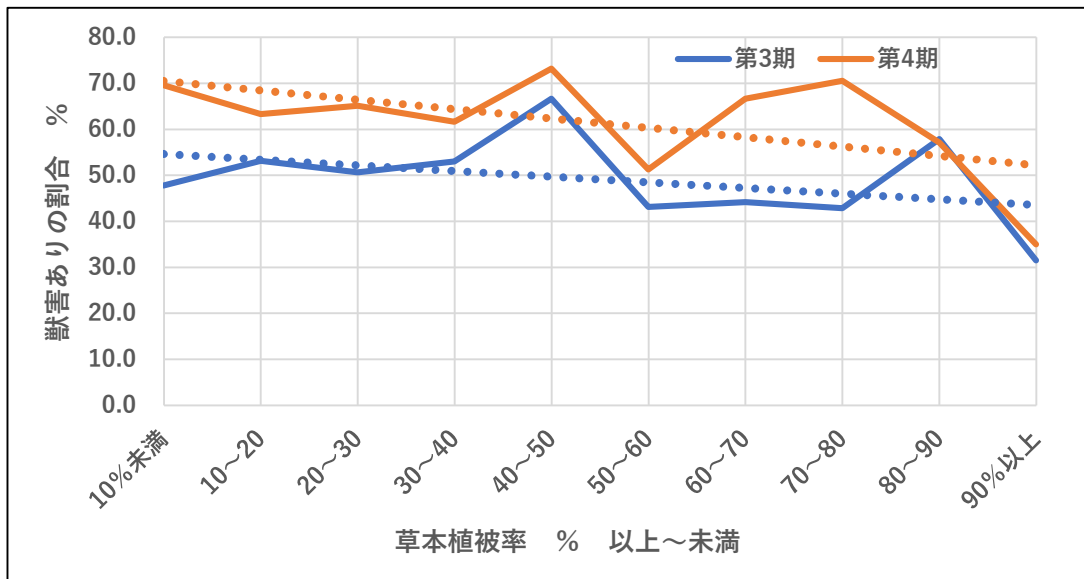
図表3-114 草本植被率別の獣害ありの割合
