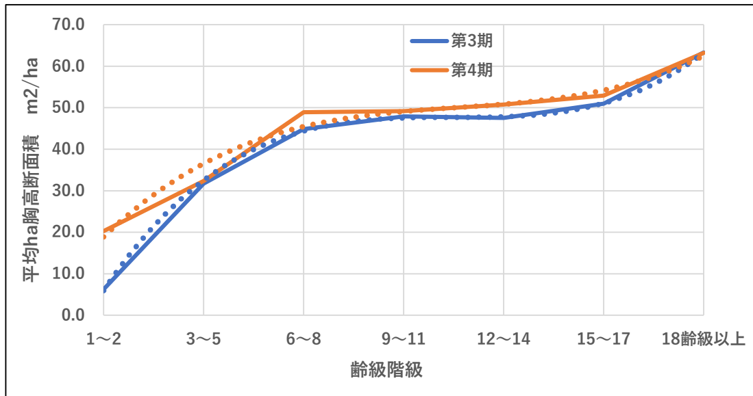
図表3-93 齢級階級別の ha 当り胸高断面積
