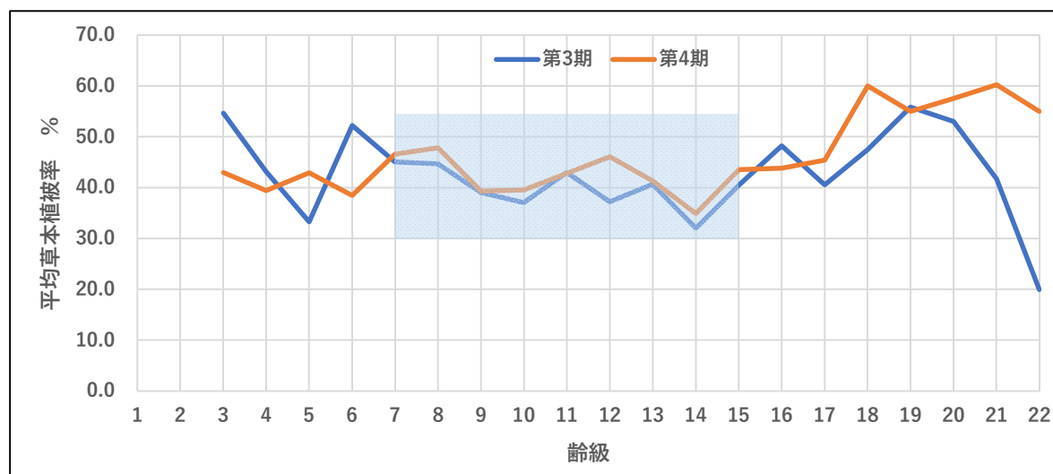
図表 5-3 齢級別の平均草本植被率
