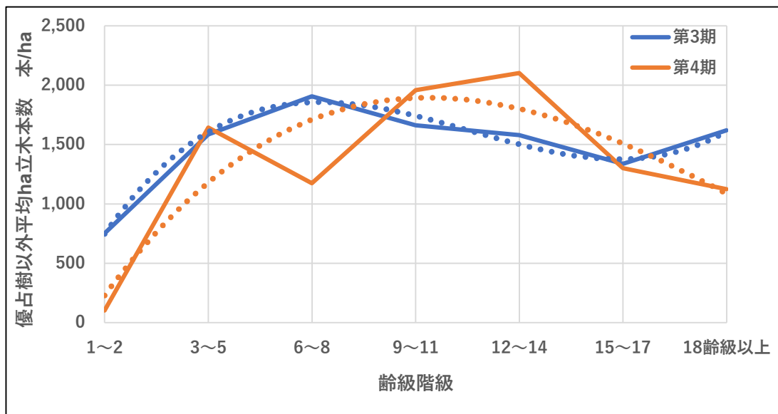
図表3-94 齢級階級別の平均 ha 当り低層木立木本数
