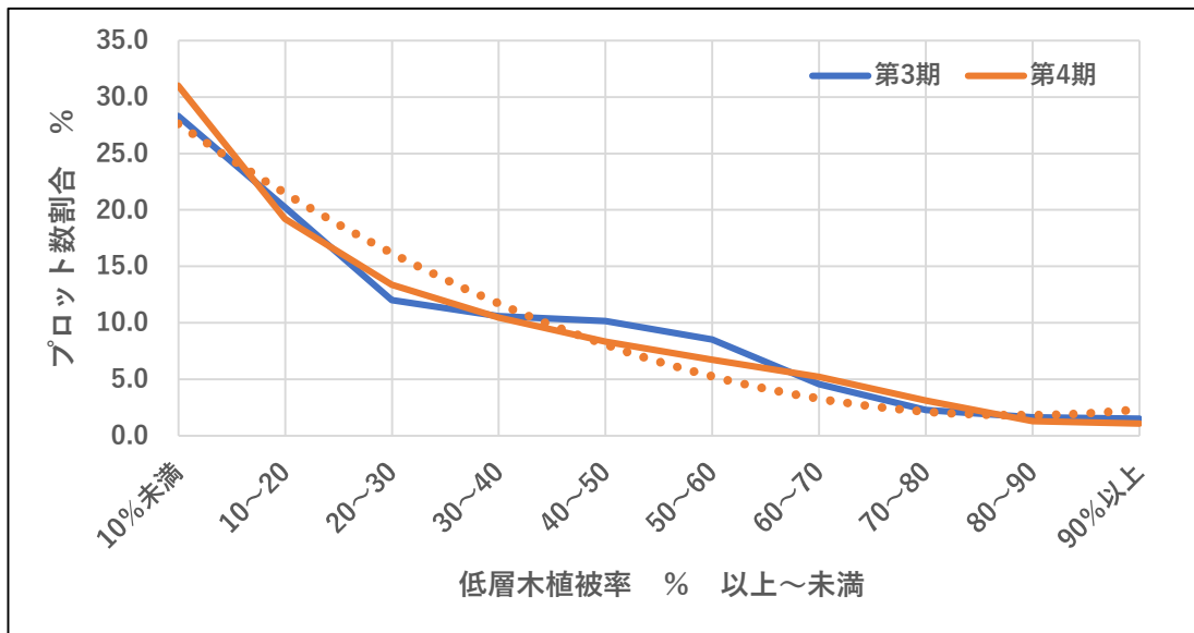
図表3-73 低層木植被率別プロット数割合
