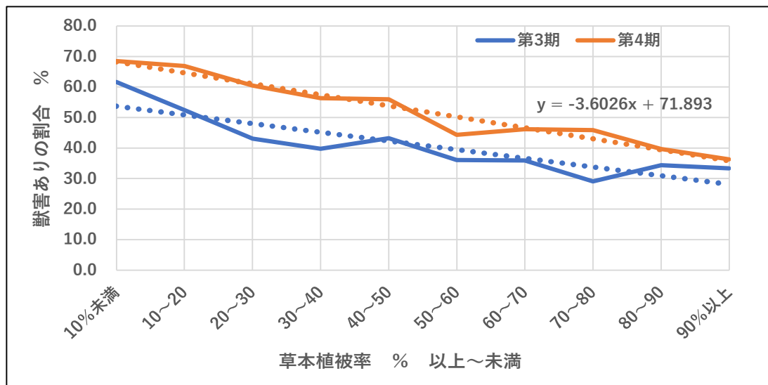
図表3－91 草本植被率別獣害ありの割合
