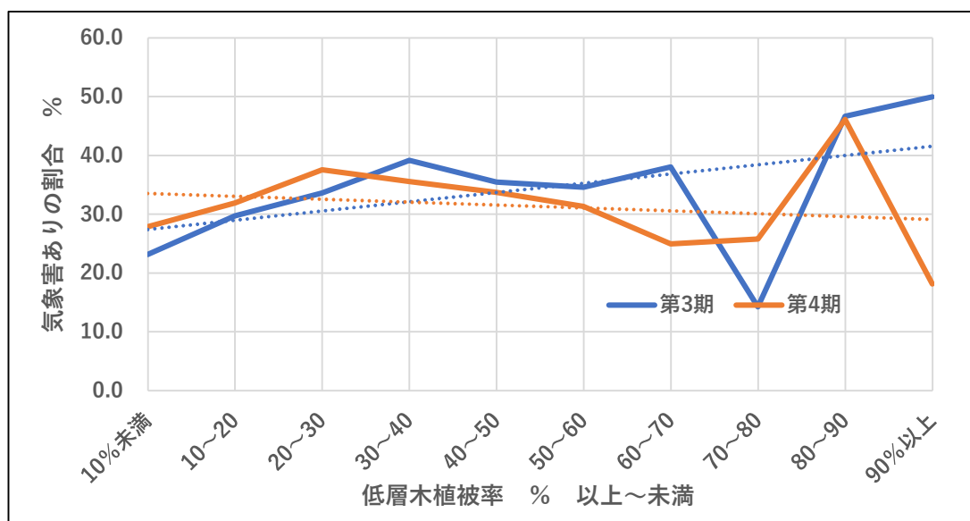
図表3-82 低層木植被率別気象害ありの割合
