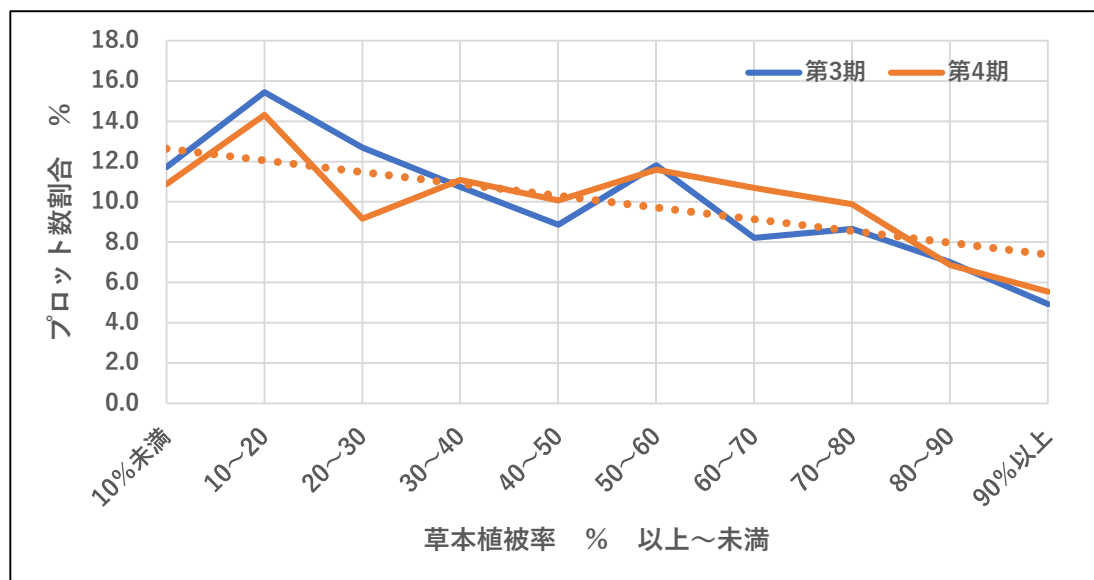
図表3-83 草本植被率別プロット数の割合
