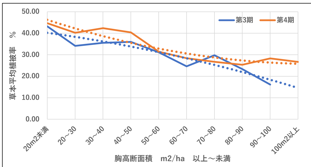
図表3-105 胸高断面積別の平均草本植被率
