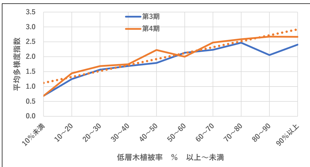
図表3-78 低層木植被率別平均シャノン・ウィナーの多様度指数
