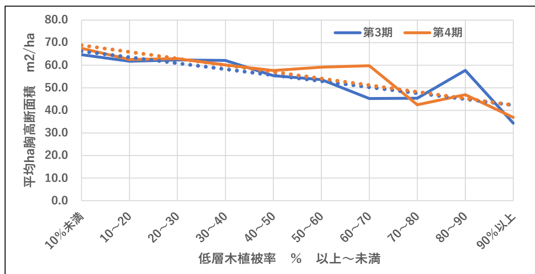
図表3-75 低層木植被率別 ha 当り平均胸高断面積
