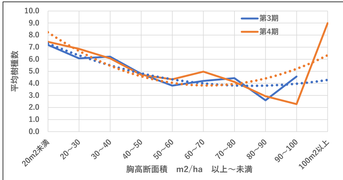
図表3-104 胸高断面積別の平均樹種数
