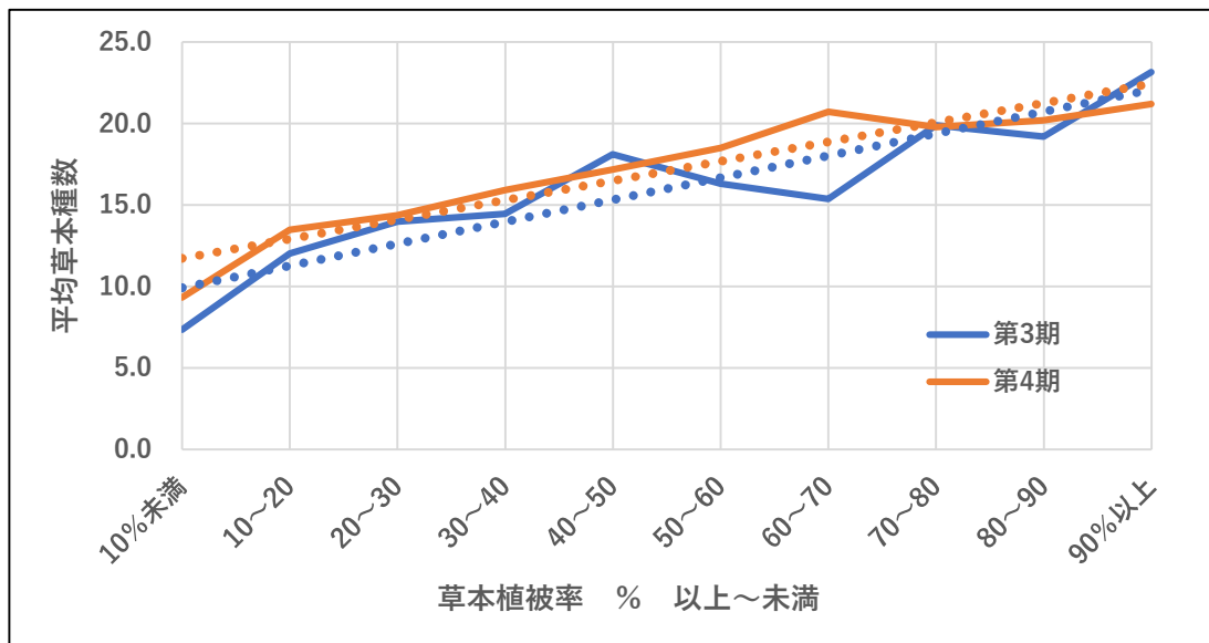
図表3－90 草本植被率別平均草本種数
