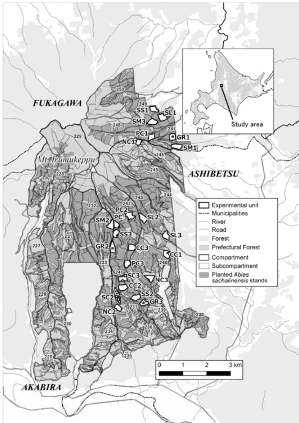
図表4-1 REFRESH プロジェクトの実証実験地全体図および実験区
