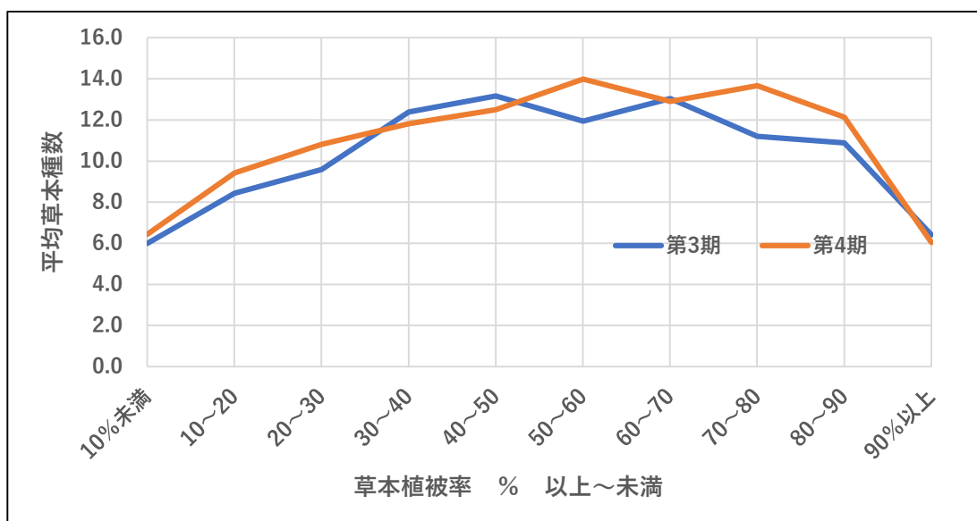
図表3-113 草本植被率別の平均草本種数
