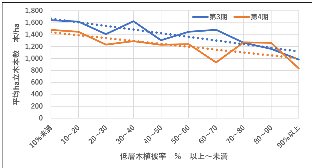
図表3-108 低層木植被率別の平均 ha 当り立木本数
