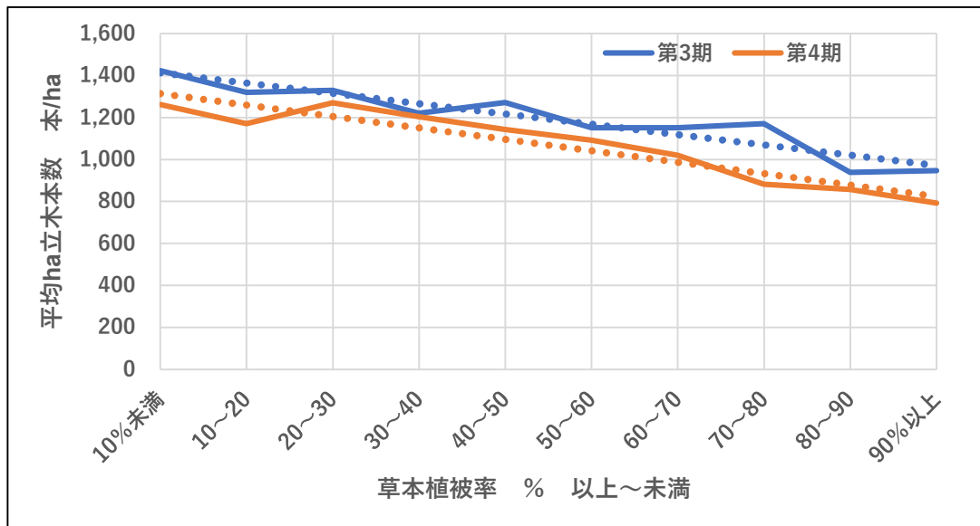
図表3－84 草本植被率別平均 ha 当り立木本数
