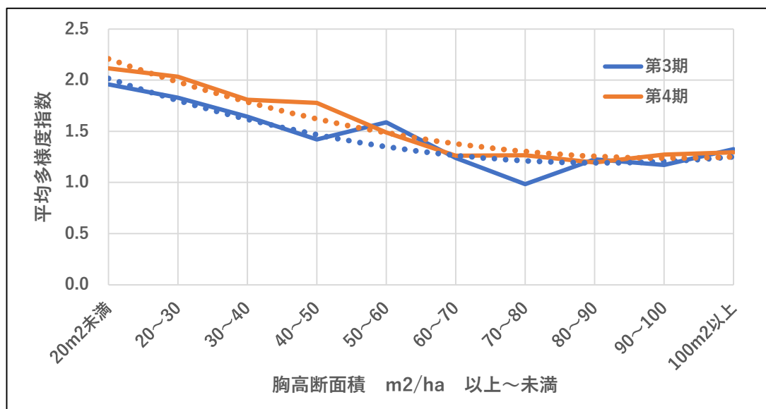
図表3-68 胸高断面積別平均シャノン・ウィナーの多様度指数
