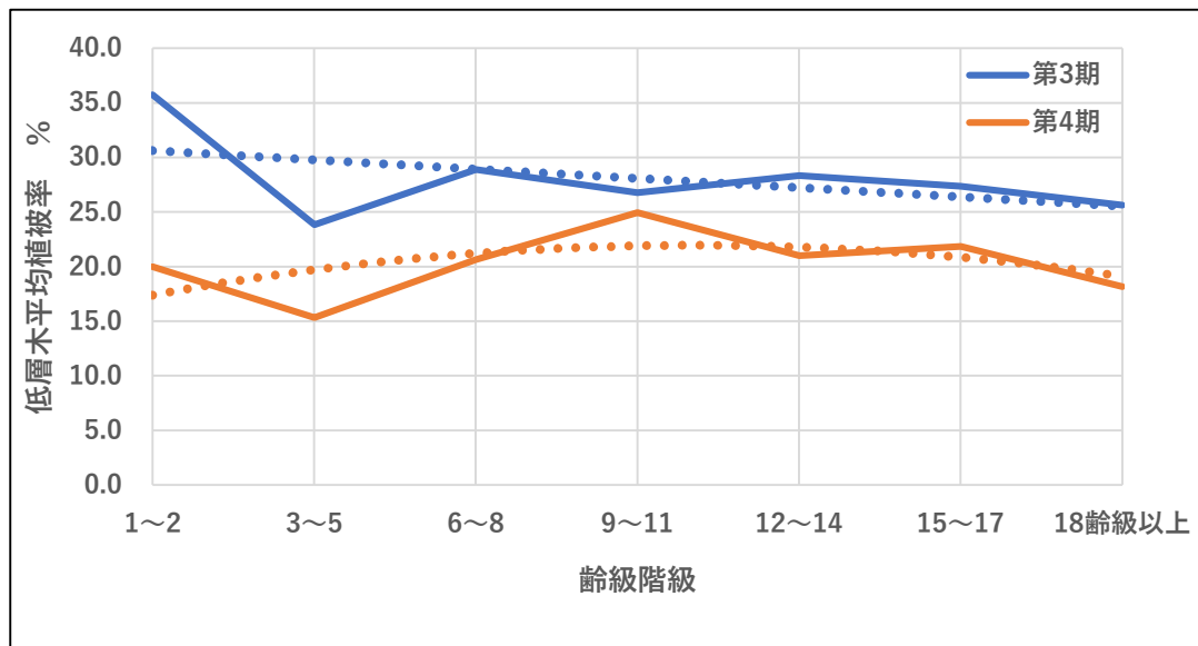
図表3－95 齢級階級別の平均低層木植被率
