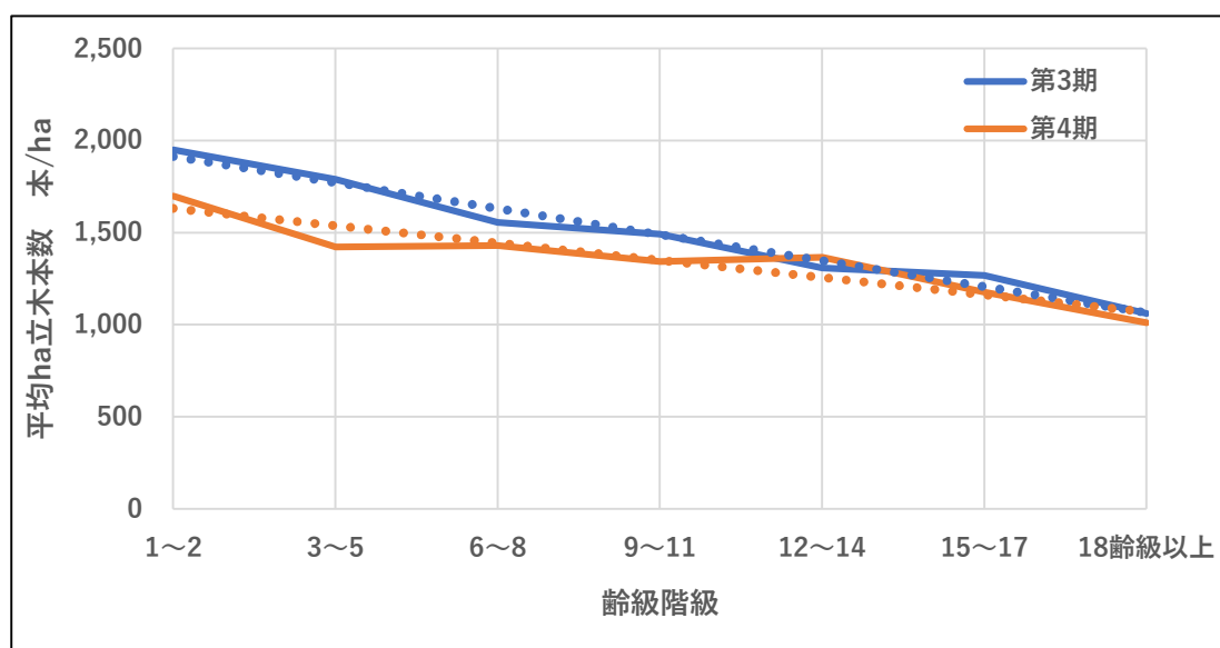
図表3-92 齢級階級別の ha 当り立木本数
