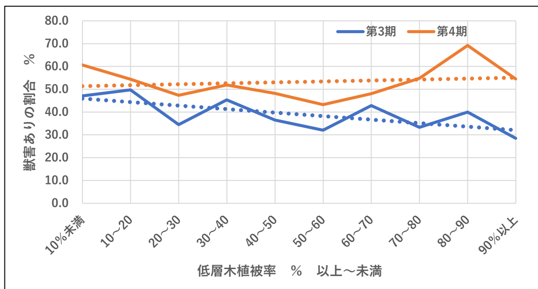
図表3-81 低層木植被率別獣害ありの割合
