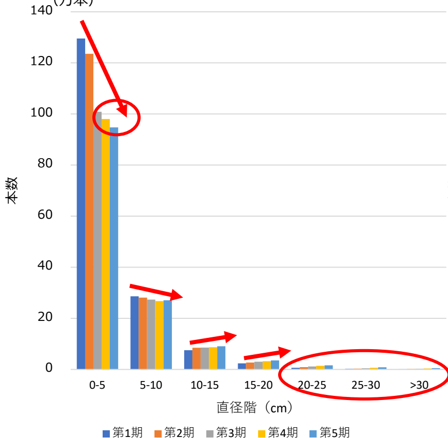
直径階別本数の時系列変化（アラカシ・全国） (万本)
