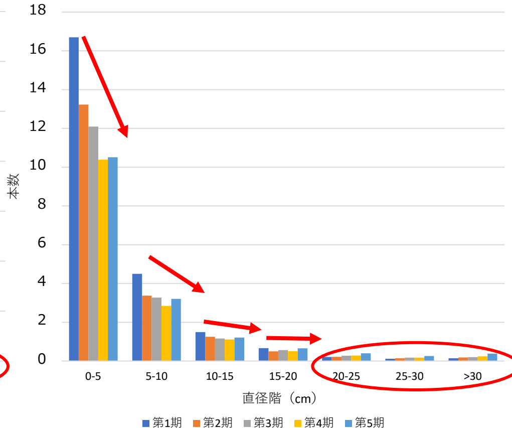
直径階別本数の時系列変化（シラカシ・全国） (万本)
