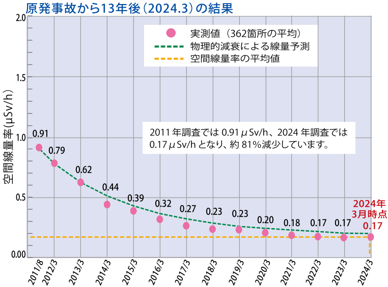
図1 放射性セシウムの物理減衰曲線とモニタリング実測値(362箇所の平均値)の関係
