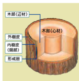
図1 樹幹の構造
