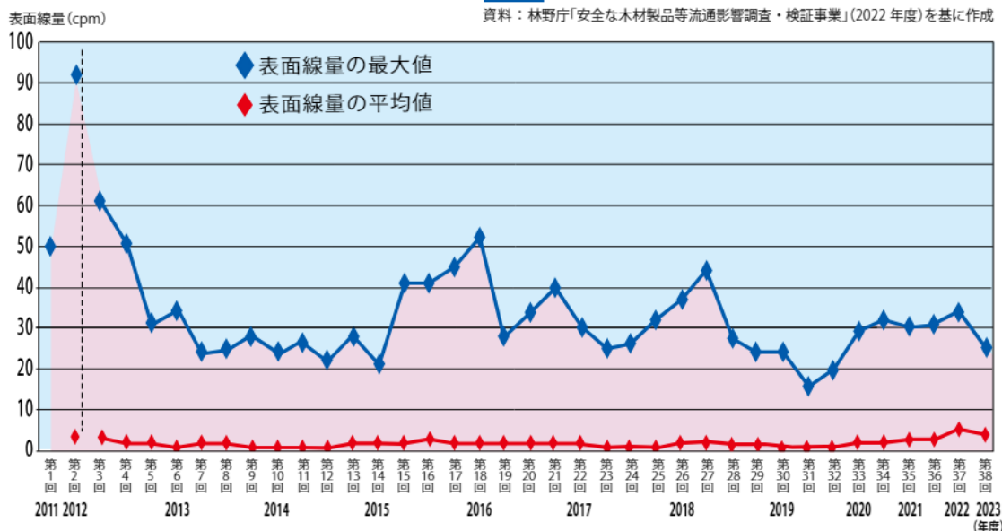
図2 製材品の表面線量
