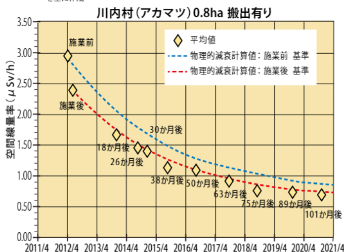
図1 森林における放射性物質対策実証(間伐等の効果)
